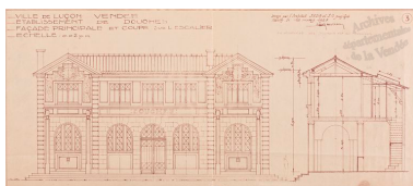
Aménagement du minage en bains-douches. Premier projet par Marcel Manceau en 1928 : façade principale et coupe sur l'escalier. Autr. Marcel Manceau, Phot. Patrice (reproduction) Giraud IVR52_20118500388NUCA
