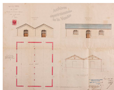
Projet de minage, non réalisé, par Léon Ballereau en 1860, par extension de la poissonnerie : projet de minage. Autr. Léon Ballereau, Phot. Patrice (reproduction) Giraud IVR52_20118500385NUCA
