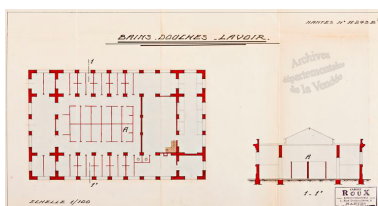
Plan et coupe au 1/100e des bains-douches par le cabinet Roux, vers 1930. Autr. Roux, Phot. Patrice (reproduction) Giraud IVR52_20118500396NUCA
