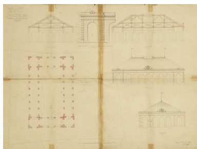
Projet réalisé, par Léon Ballereau, le 1er juillet 1865. Autr. Léon Ballereau, Phot. Patrice (reproduction) Giraud IVR52_20068500139NUCA
