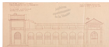
Aménagement du minage en bains-douches. Premier projet par Marcel Manceau en 1928 : façade latérale. Autr. Marcel Manceau, Phot. Patrice (reproduction) Giraud IVR52_20118500390NUCA
