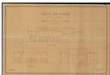
Aménagement du minage en bains-douches. Coupes par Perreau, architecte, vers 1930. Autr. Perreau IVR52_20098500025NUCA
