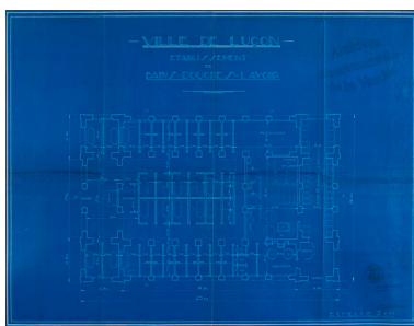
Aménagement du minage en bains-douches. Plan par Perreau, architecte, vers 1930. Autr. Perreau, Phot. Patrice (reproduction) Giraud IVR52_20118500391NUCA
