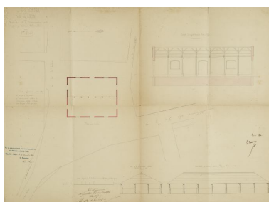
Projet de minage, non réalisé, par Léon Ballereau en 1860, par extension de la poissonnerie : état actuel de la poissonnerie. Autr. Léon Ballereau, Phot. Patrice (reproduction) Giraud IVR52_20068500138NUCA
