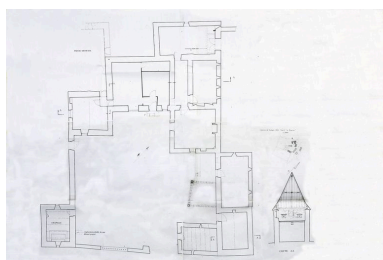
Relevé, 1989 : plan du rez-de-chaussée du logis et coupe de la chapelle. Autr. G. Coulonnier, Autr. J. Guérin, Phot. François Lasa IVR52_20085302296NUCA
