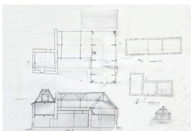
Relevé, 1989 : plan du comble et coupe longitudinale du logis, plan des dépendances sud et est. Autr. G. Coulonnier, Autr. J. Guérin, Phot. François Lasa IVR52_20085302297NUCA
