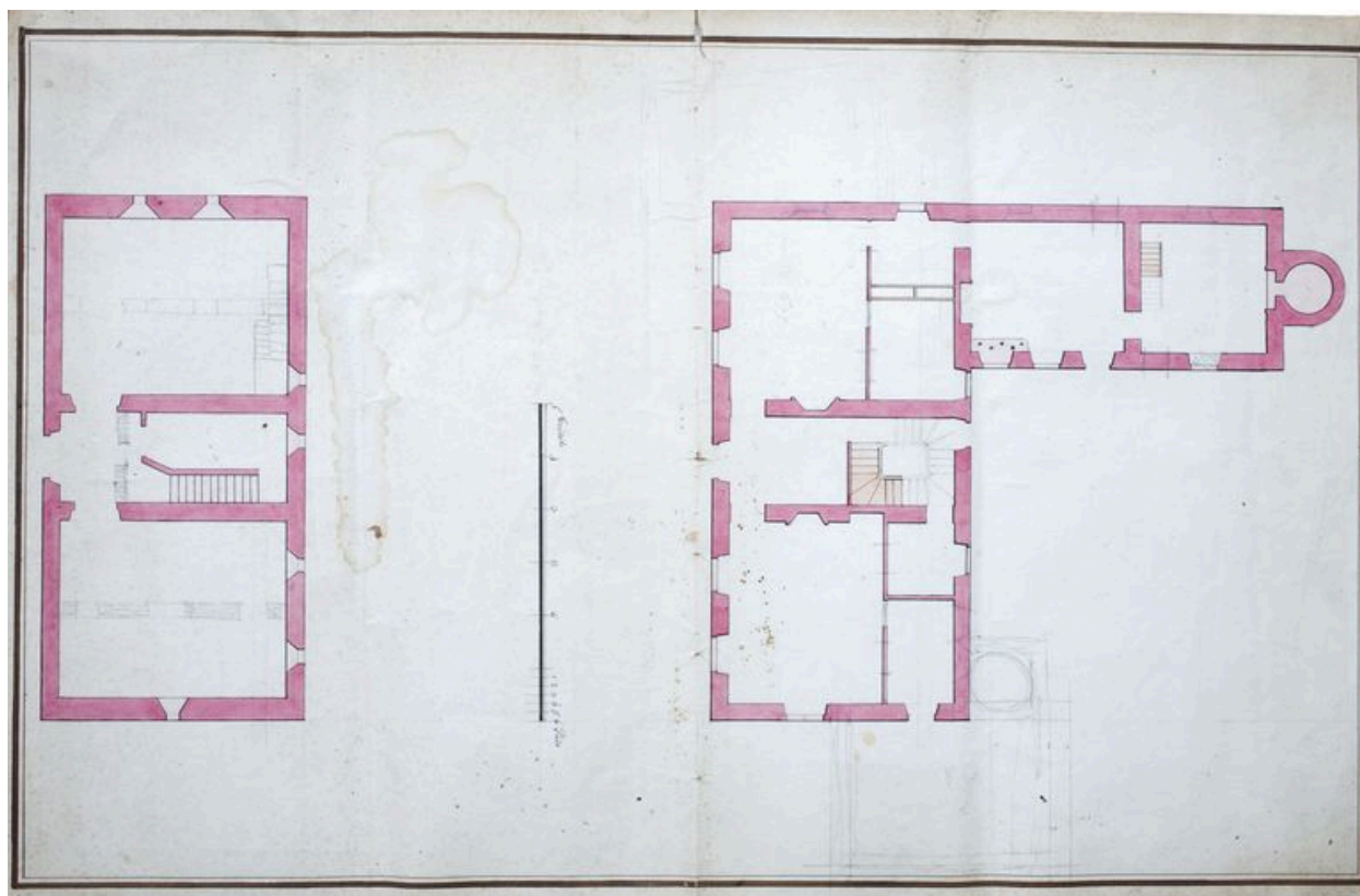
Plan du sous-sol et du rez-de-chaussée du château, vers 1830.
