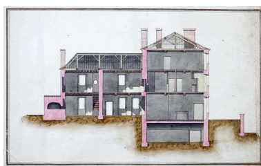
Coupe transversale du château, vers 1830. Repro. Yves Guillotin IVR52_20095300425NUCA
