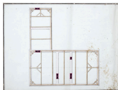
Plan des combles du château, vers 1830. Repro. Yves Guillotin IVR52_20095300428NUCA
