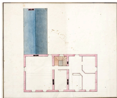
Plan du deuxième étage du château, vers 1830. Repro. Yves Guillotin IVR52_20095300427NUCA
