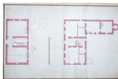
Plan du sous-sol et du rez-de-chaussée du château, vers 1830. Repro. Yves Guillotin IVR52_20095300422NUCA
