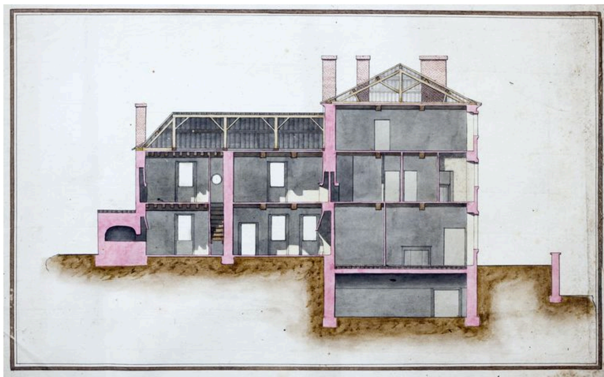
Coupe transversale du château, vers 1830.
