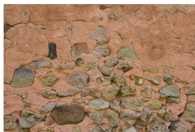
Le Petit Verger, étable. Maçonnerie de moellons enduits à chaux et sable ferrugineux des carrières de Sables (La Davière). Phot. Yves Guillotin IVR52_20117200553NUCA
