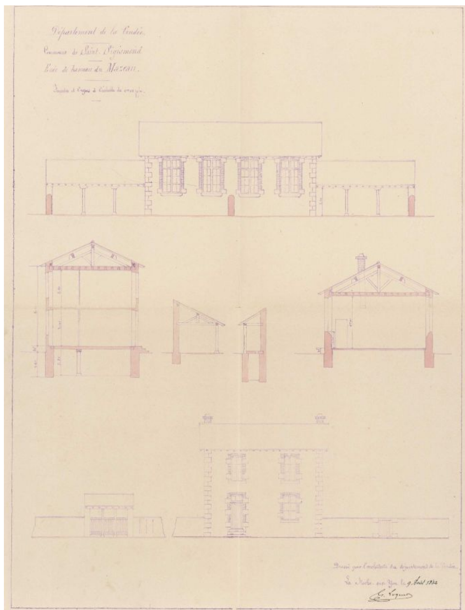
Projet d'école de hameau au Mazeau par Georges Loquet, 9 août 1882 : élévations et coupes.
