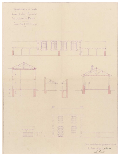
Projet d'école de hameau au Mazeau par Georges Loquet, 9 août 1882 : élévations et coupes. Repro. Yannis Suire IVR52_20238500274NUCA
