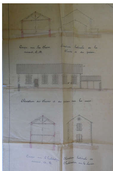
Projet de classe enfantine et d'aménagement de la mairie et du logement, par Abel Filuzeau, 1er avril 1890 : élévation et coupes des classes et du préau d'une part, de la mairie-logement d'autre part. Repro. Yannis Suire IVR52_20238500333NUCA
