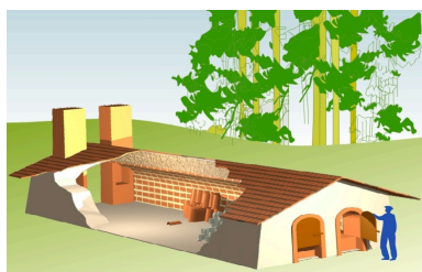
Schéma d'un four horizontal ou four couché. Dess. Zoé Lambert IVR54_20070000012NUD
