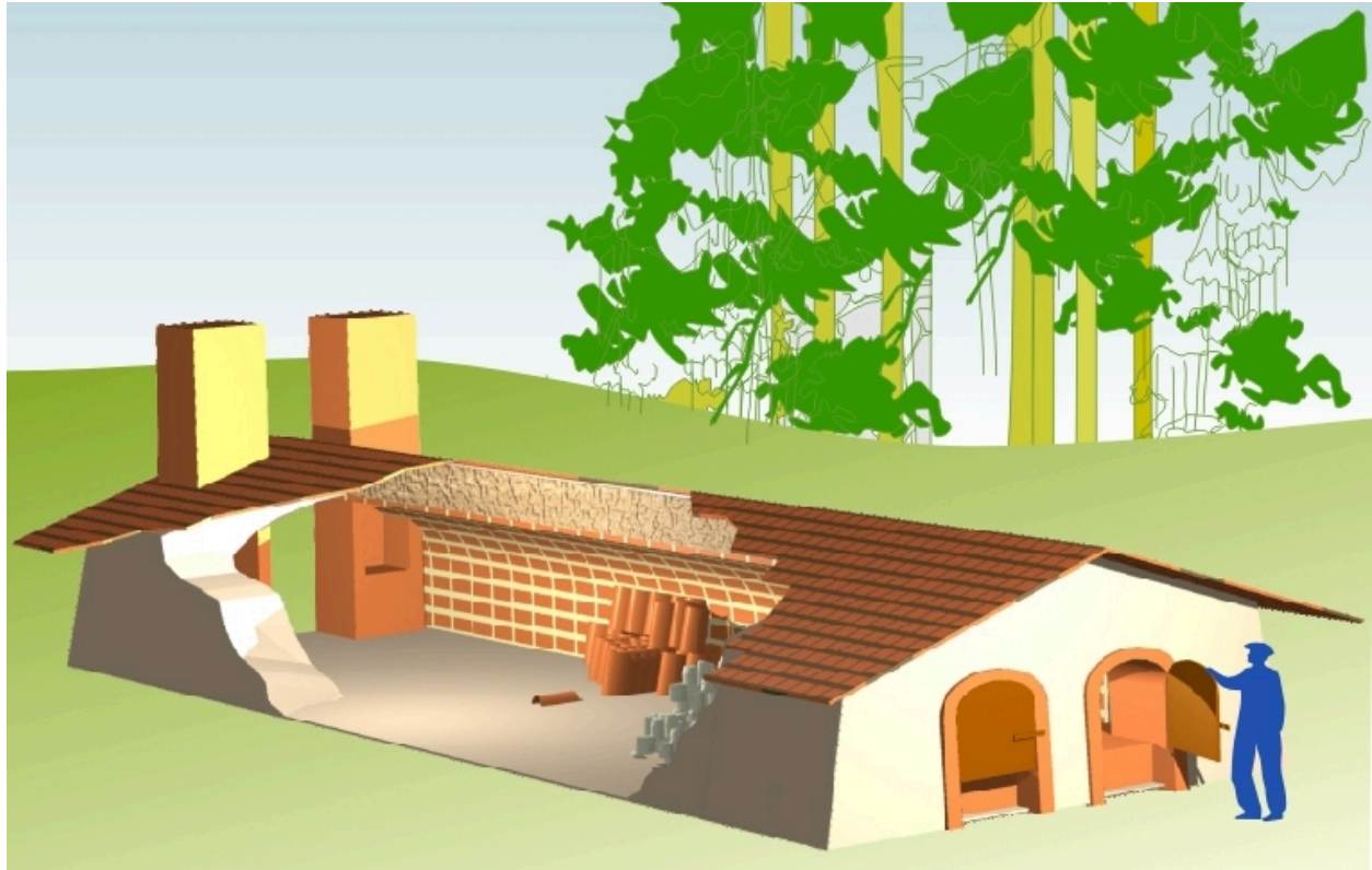
Schéma d'un four horizontal ou four couché.
