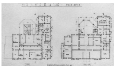
Plans du sous-sol et de l'étage au 1/100e de la mairie annexe en 1931. Autr. Paul-Henri Datessen, Phot. Denis (reproduction) Pillet IVR52_20004401253X
