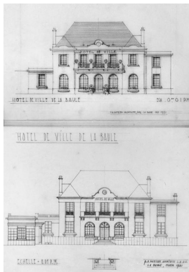
Projets de façade au 1/100e de la mairie annexe en 1931.
