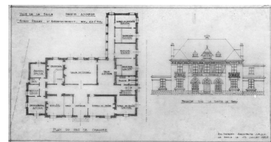
Plan du rez-de-chaussée et de la façade au 1/100e de la mairie annexe en 1928.
