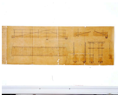
Projet d'écluse des Communes : plan, élévation et coupes de la passerelle. Autr. Charles Dupuy, Phot. François (reproduction) Lasa IVR52_20025300108XA
