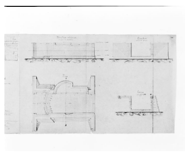
Projet d'écluse des Communes : plan, élévation et coupes. Autr. Charles Dupuy, Phot. François (reproduction) Lasa IVR52_20025300104X
