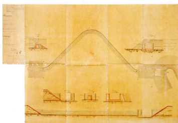
Projet de barrage des Communes : plan, élévation et coupes du barrage et du pertuis. Phot. Charles Dupuy, Phot. François (reproduction) Lasa IVR52_20025300100XA
