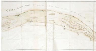
Carte géométrique d'une partie du cours de la rivière de Loire, par Magin et Blaveau, 1757, détail. Autr. Magin, Autr. Blaveau, Phot. François Lasa IVR52_20054400369NUCA
