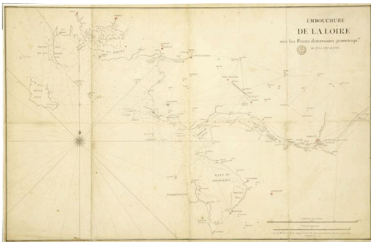
Embouchure de la Loire avec les points déterminés géométriquement en 1735, 1737 et 1738.
