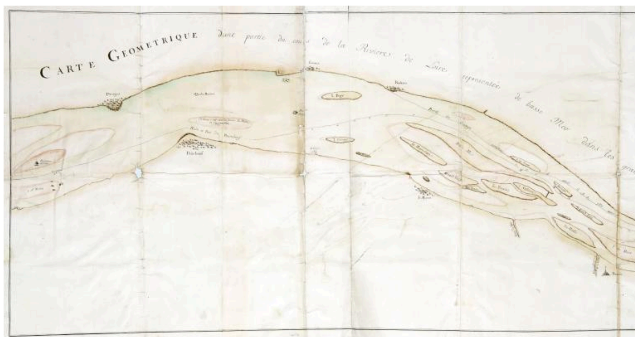
Carte géométrique d'une partie du cours de la rivière de Loire, par Magin et Blaveau, 1757, détail.
