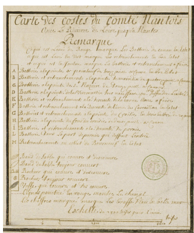
Carte des côtes du comté de Nantes et de la Loire jusqu'à Nantes, avec le report des batteries et des retranchements, [1750], détail de la légende. Phot. François Lasa IVR52_20054400797NUCA
