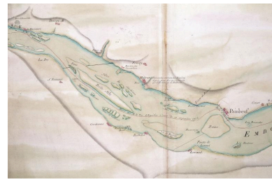
Carte figurée de la rivière de Loire pour servir au projet de rétablissement de la navigation, [1764], détail. Phot. Patrice (reproduction) Giraud IVR52_19954400594XA
