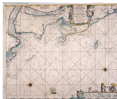
Carte marine, par Wooght, 2e moitié XVIIe siècle. Autr. Wooght, Phot. Bernard (reproduction) Renoux IVR52_19928500099VA
