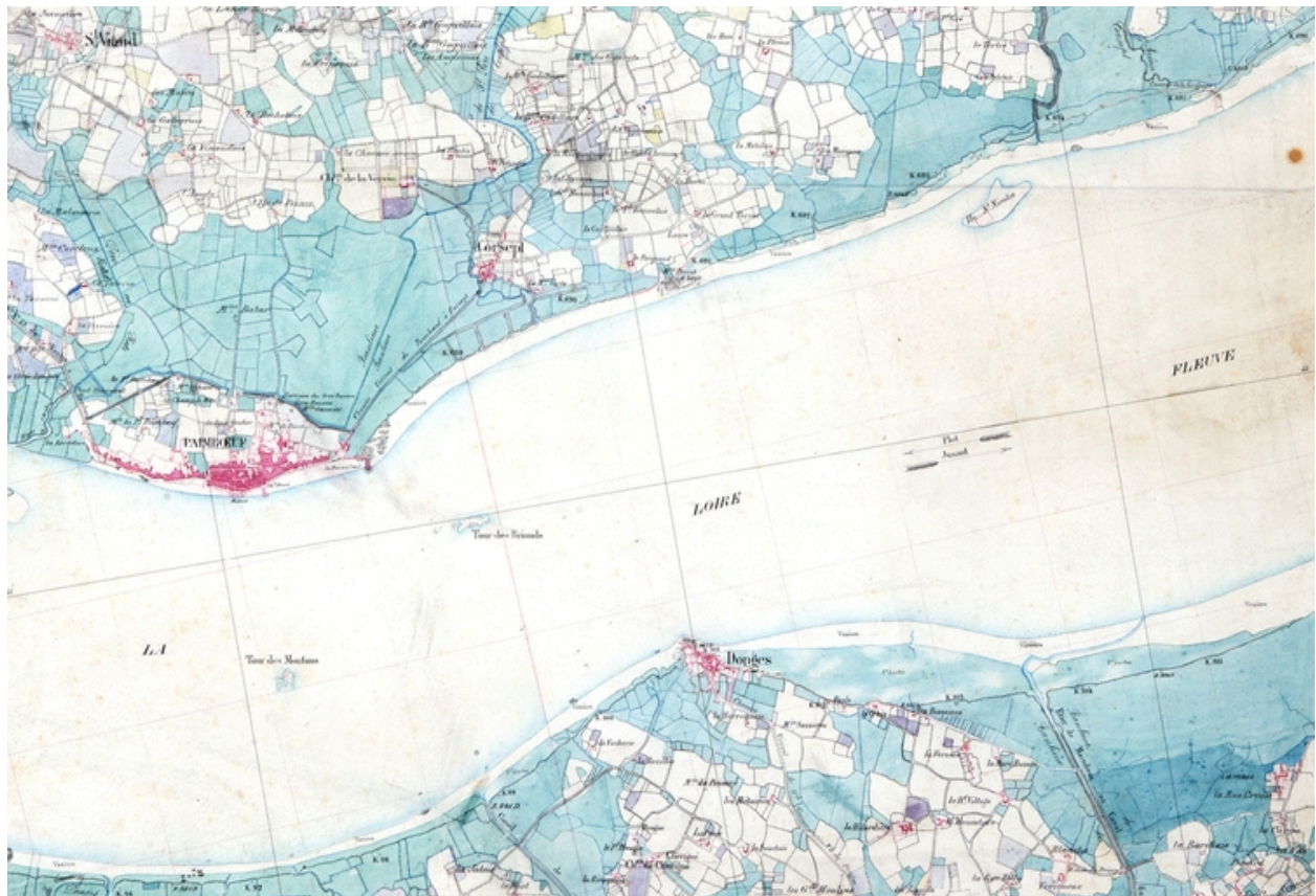
Carte topographique de la Loire dite de Coumes, 1863, détail.
