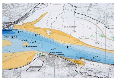
Carte générale de la Loire maritime, fonds IGN avec le report des données du Port autonome, 1984, détail. Phot. François Lasa IVR52_20084400401NUCA
