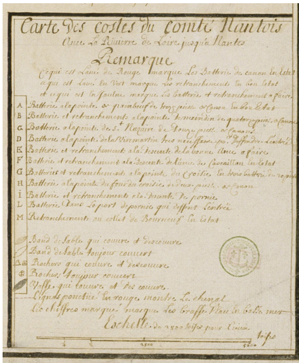
Carte des côtes du comté de Nantes et de la Loire jusqu'à Nantes, avec le report des batteries et des retranchements, [1750], détail de la légende.
