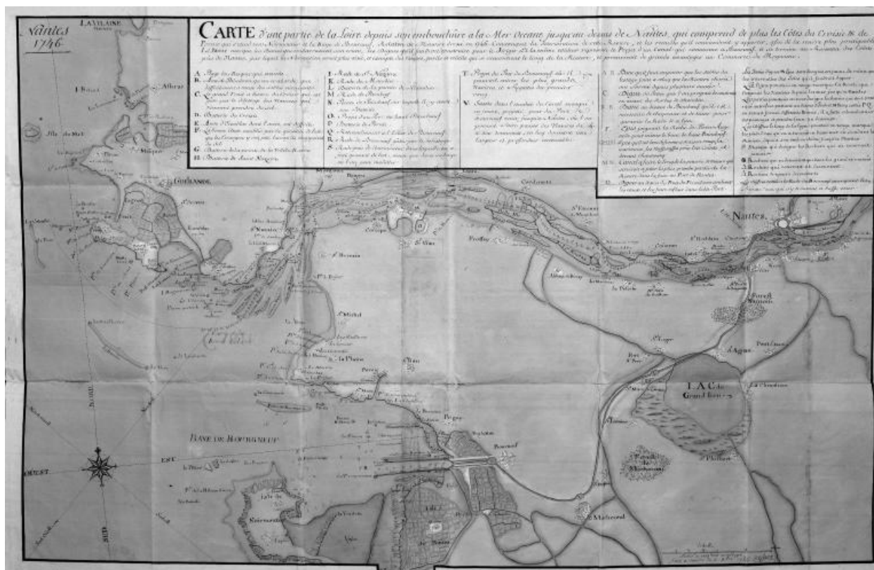
Carte de l'embouchure de la Loire par Decaux, avec un projet de port à Paimboeuf et celui d'un canal entre Bourgneuf et le ruisseau des Couëts près de Nantes, 1746.
