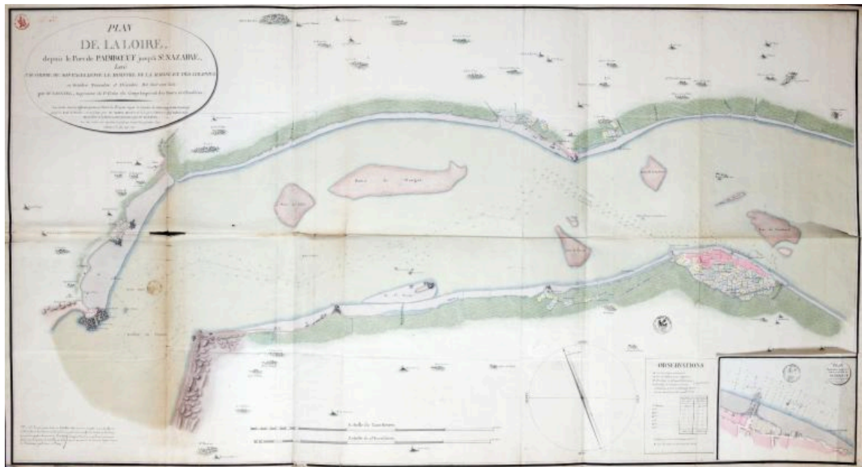
Plan de la Loire de Paimboeuf à Saint-Nazaire, par Rapatel, 1808.
