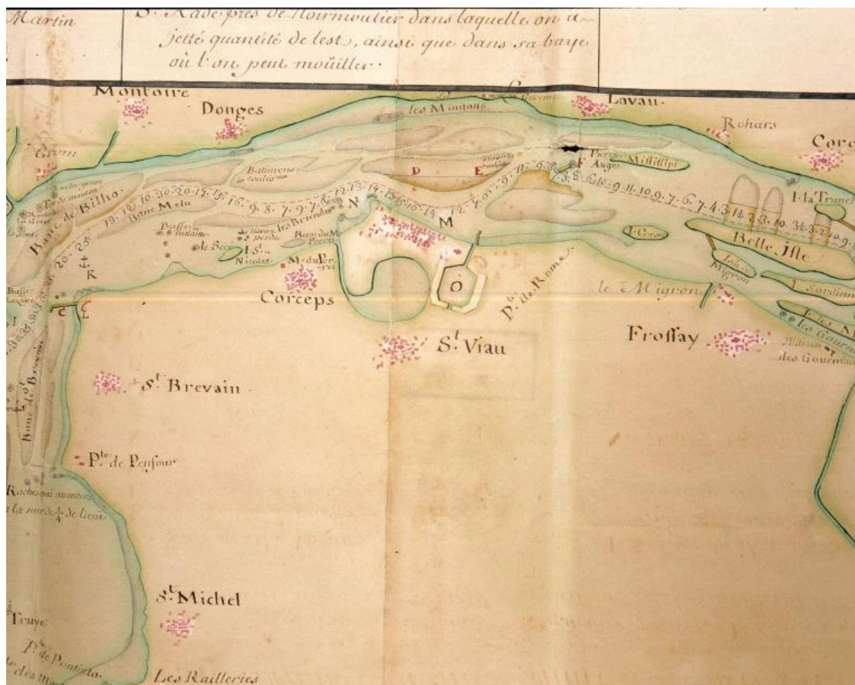
Carte de l'embouchure de la Loire par Decaux, avec un projet de port à Paimboeuf et celui d'un canal entre Bourgneuf et le ruisseau des Couëts près de Nantes, 1746, détail du port de Paimboeuf.
