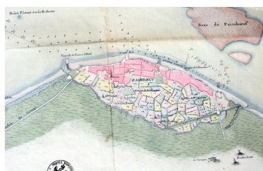
La Loire entre le Migron et Paimbœuf, carte actualisée en 1812 d'après une carte établie en 1757 par Magin, détail. Autr. Magin, Phot. François Lasa IVR52_20054400333NUCA
