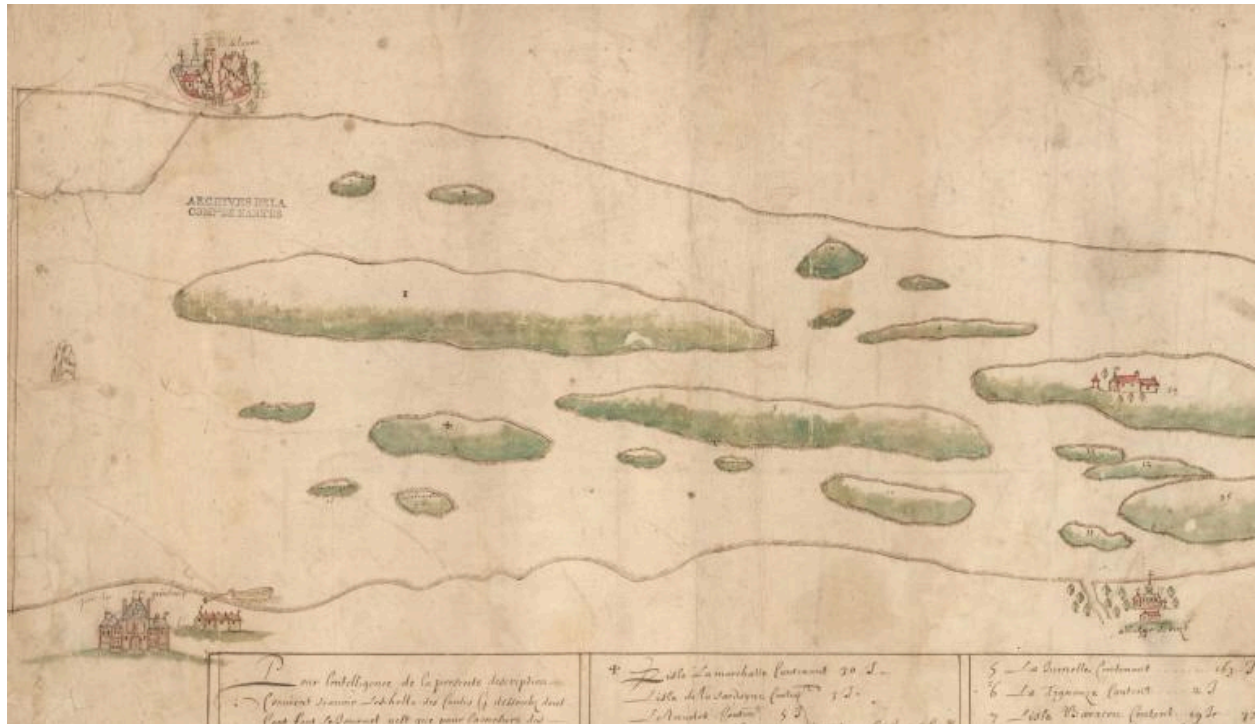
Carte d'arpentage des îles de la Loire depuis Ingrandes jusqu'à Paimboeuf, par Brion, 1665, détail : l'extrémité ouest entre Lavau et Paimboeuf.
