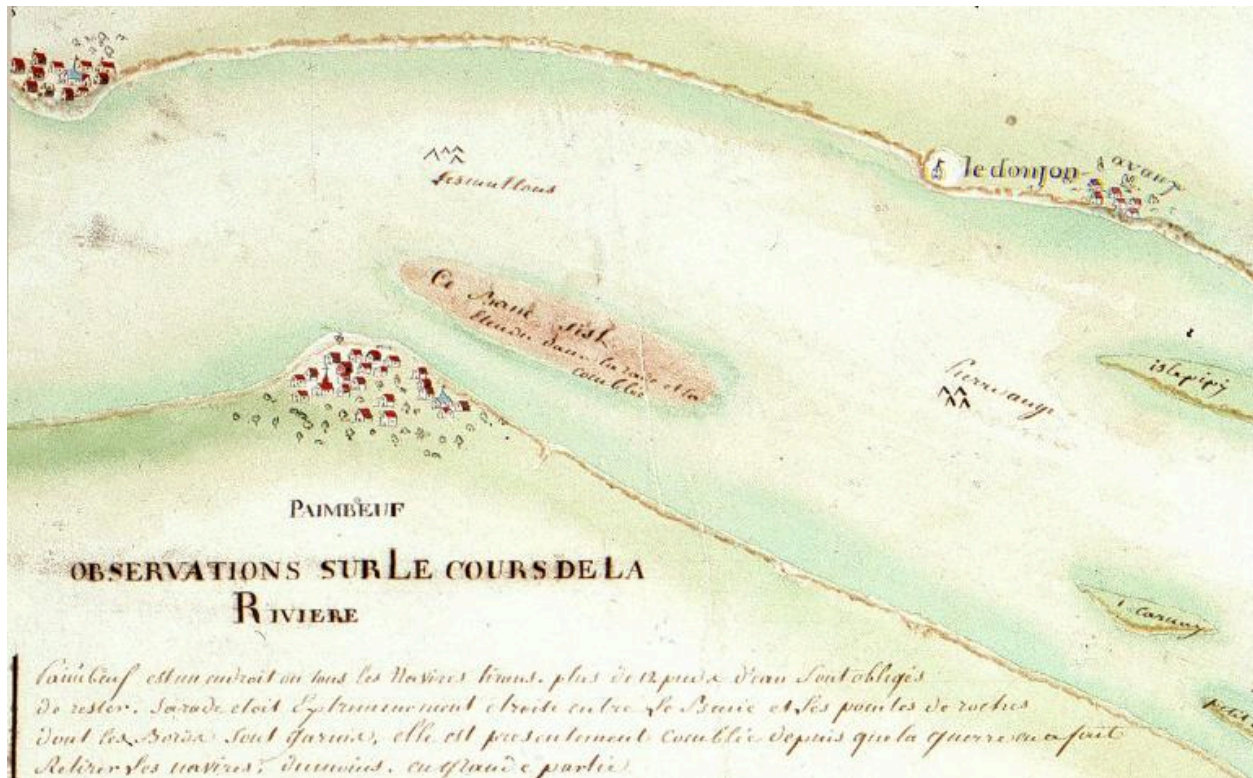
Carte de l'embouchure de la Loire commentée, [1770], détail : le port de Paimboeuf.
