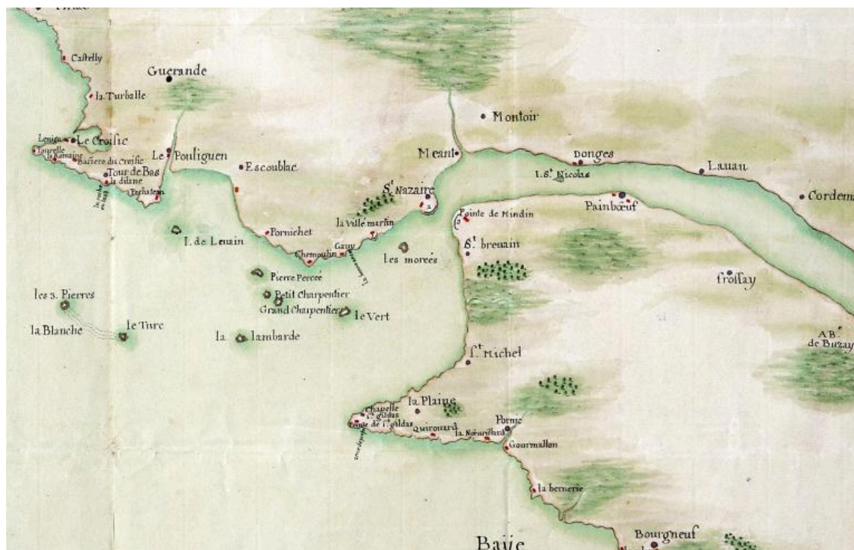
Carte des côtes du comté de Nantes avec report des corps de garde, par Touros, 1744, détail.
