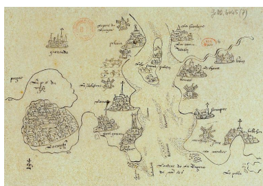
Carte de l'embouchure de la Loire, par Jean Alfonse, 1545. Phot. Bernard (reproduction) Gil, Autr. Jean Alfonse IVR52_20094401272NUCA
