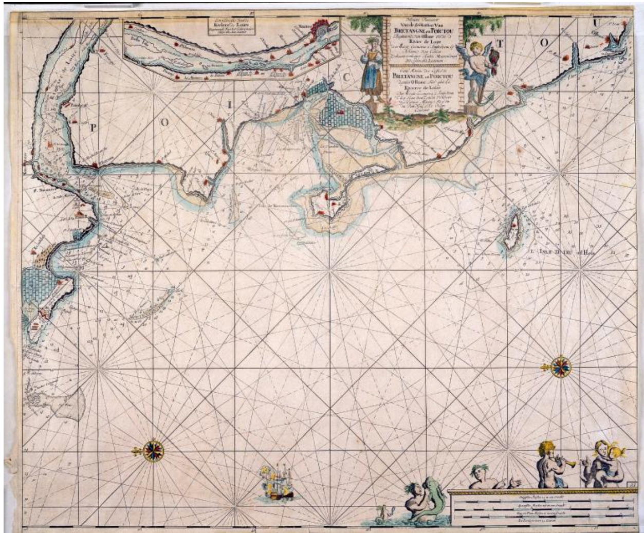
Carte marine, par Wooght, 2e moitié XVIIe siècle.
