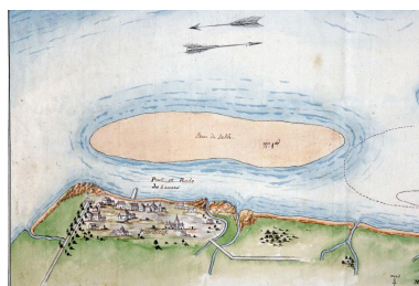
La Loire entre le Migron et Paimbœuf, carte actualisée en 1812 d'après une carte établie en 1757 par Magin, détail. Autr. Magin, Phot. François Lasa IVR52_20054400333NUCA
