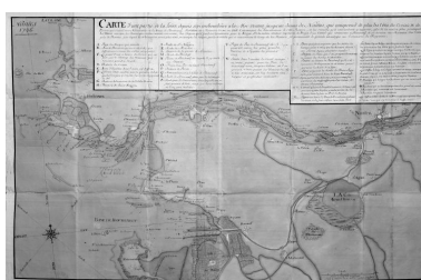
Carte de l'embouchure de la Loire par Decaux, avec un projet de port à Paimboeuf et celui d'un canal entre Bourgneuf et le ruisseau des Couëts près de Nantes, 1746. Autr. Decaux, Phot. Patrice (reproduction) Giraud IVR52_19954400570V
