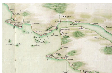
Carte des côtes du comté de Nantes avec report des corps de garde, par Touros, 1744, détail. Autr. Touros, Phot. François Lasa IVR52_20074400013NUCA
