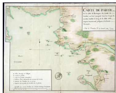
Carte des côtes du comté de Nantes avec report des corps de garde, par Touros, 1744. Autr. Touros, Phot. François Lasa IVR52_20054400339NUCA
