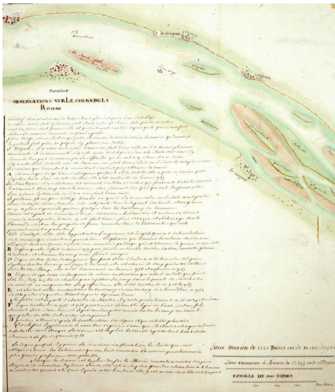
Carte de l'embouchure de la Loire liée à des observations précises sur son cours, [1770], détail.
