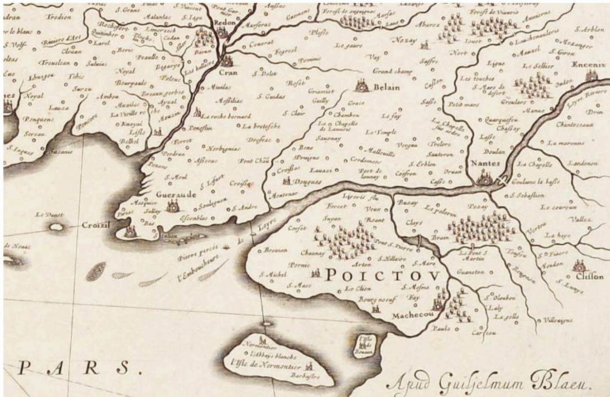
Carte du duché de Bretagne, par Blaeu, [1635], détail.
