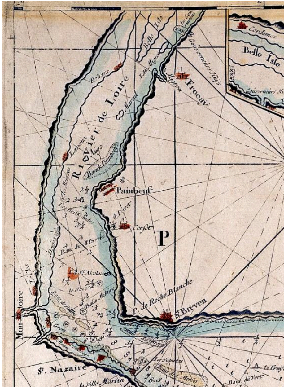
Carte marine, par Wooght, 2e moitié XVIIe siècle, détail.
