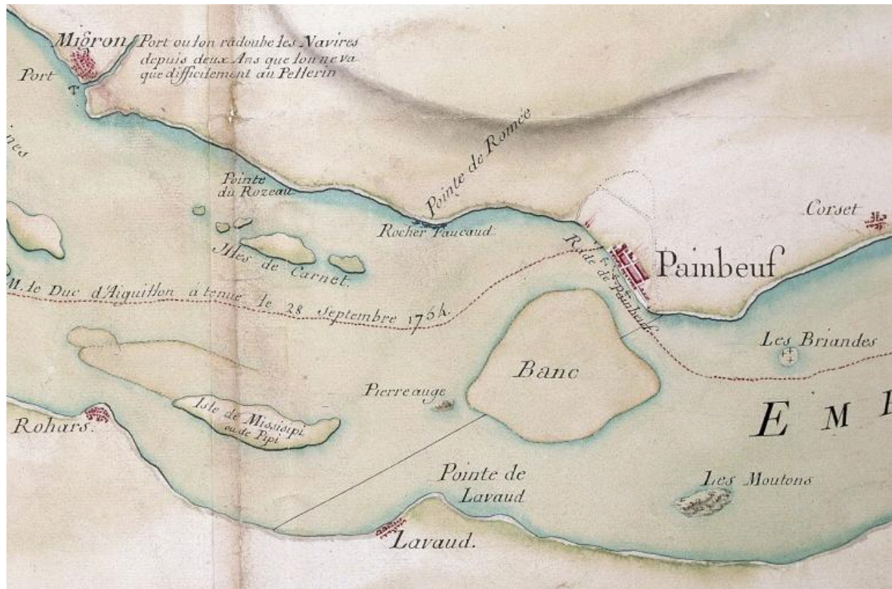
Carte figurée de la rivière de Loire pour servir au projet de rétablissement de la navigation, 1764, détail.
