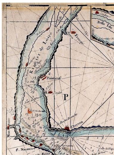
Carte marine, par Wooght, 2e moitié XVIIe siècle, détail. Autr. Wooght, Phot. Bernard (reproduction) Renoux IVR52_19928500163NUCA
