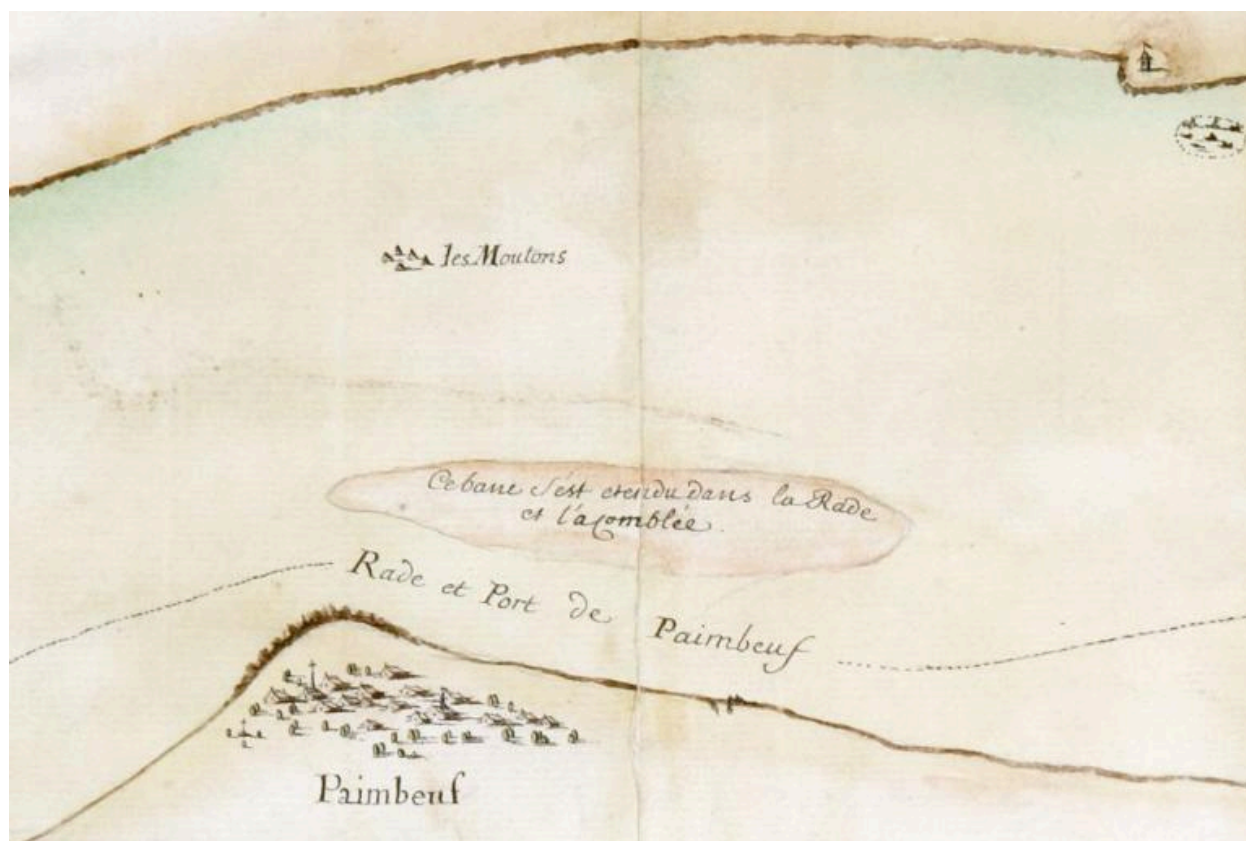
Carte géométrique d'une partie du cours de la rivière de Loire, par Magin et Blaveau, 1757, détail.
