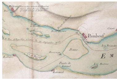
Carte figurée de la rivière de Loire pour servir au projet de rétablissement de la navigation, 1764, détail. Phot. François Lasa IVR52_20114400675NUCA
