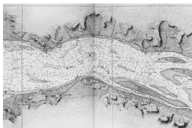
Cours de la Loire depuis Nantes jusqu'à son embouchure levée en 1821, par les ingénieurs hydrographes de la marine, 1828. Autr. C.-F. Beutemps-Beaupré IVR52_20054400795NUCA
