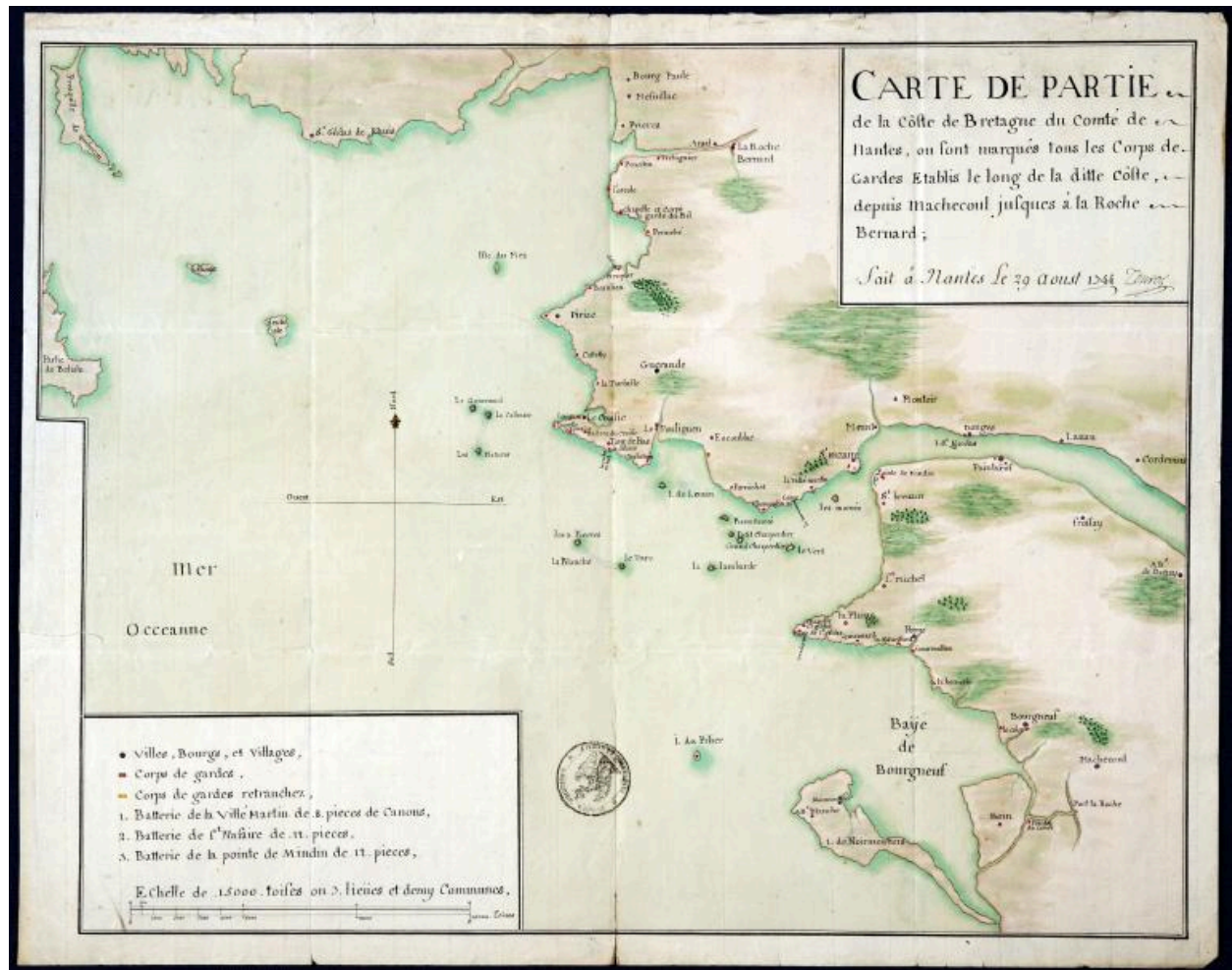
Carte des côtes du comté de Nantes avec report des corps de garde, par Touros, 1744.
