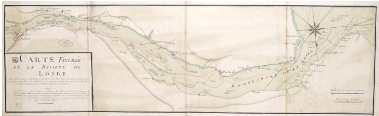
Carte figurée de la rivière de Loire pour servir au projet de rétablissement de la navigation, [1764].
