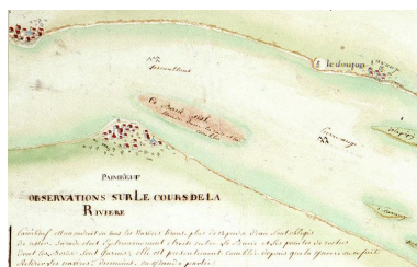
Carte de l'embouchure de la Loire commentée, [1770], détail : le port de Paimbœuf. Phot. Patrice (reproduction) Giraud IVR52_20114400674NUCA
