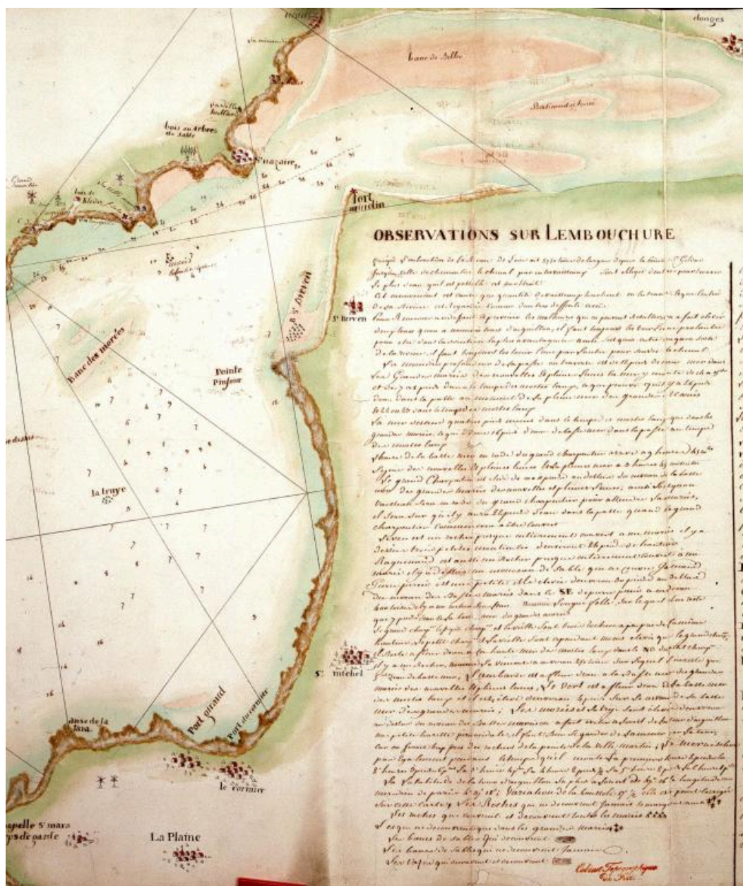
Carte de l'embouchure de la Loire liée à des observations précises sur son cours, [1770], détail.
