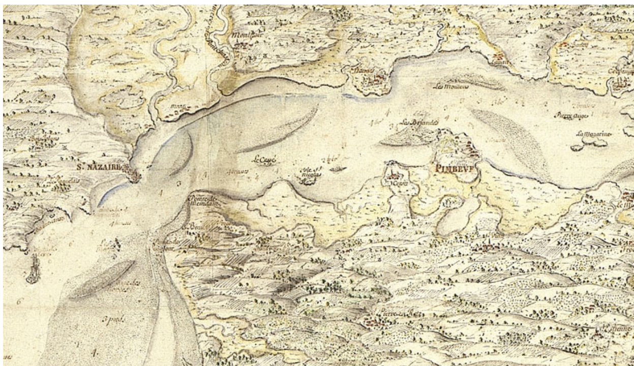
Carte topographique des entrées et cours de la rivière de Loyre et de celles qui s'y dégorgent () par Louis de Clerville, [1670], détail.
