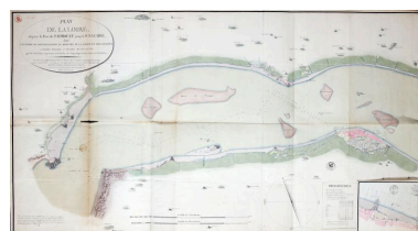
Plan de la Loire de Paimbœuf à Saint-Nazaire, par Rapatel, 1808. Autr. Rapatel, Phot. François Lasa IVR52_20054400344NUCA
