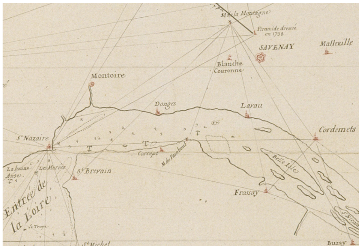
Embouchure de la Loire avec les points déterminés géométriquement en 1735, 1737 et 1738, détail.
