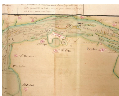
Carte de l'embouchure de la Loire par Decaux, avec un projet de port à Paimboeuf et celui d'un canal entre Bourgneuf et le ruisseau des Couëts près de Nantes, 1746, détail du port de Paimboeuf. Autr. Decaux, Phot. Patrice (reproduction) Giraud IVR52_19954400602XA
