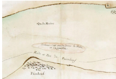
Carte géométrique d'une partie du cours de la rivière de Loire, par Magin et Blaveau, 1757, détail. Autr. Magin, Autr. Blaveau, Phot. François Lasa IVR52_20054400370NUCA
