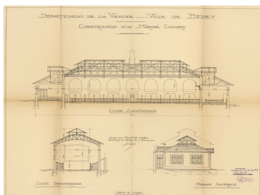
Projet de marché couvert par Abel Filuzeau, 5 décembre 1922 : coupes et élévation latérale. Repro. Yannis Suire IVR52_20238502280NUCA
