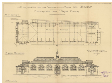
Projet de marché couvert par Abel Filuzeau, 5 décembre 1922 : plan et élévation principale. Repro. Yannis Suire IVR52_20238502279NUCA
