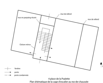
Plan schématique de la cage d'escalier au rez-de-chaussée. Dess. Frédéric Dufrêche IVR52_20074403092NUD
