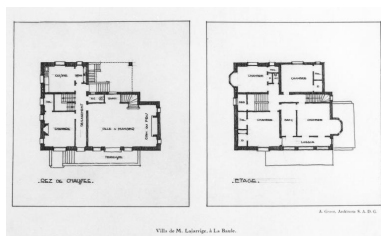
Plans du rez-de-chaussée et de l'étage de la villa Kenavo. Autr. Adrien Grave, Phot. Denis (reproduction) Pillet IVR52_19984400591X
