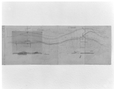
Plan d'ensemble du site extrait du plan parcellaire des bords de la Mayenne à canaliser entre Sacé et le pont de Montgiroux : anciens barrage et moulin (détruits), premier projet de barrage à écluse (non réalisé), deuxième projet (réalisé) en aval. Autr. Charles Dupuy, Repro. François Lasa IVR52_20025300264X
