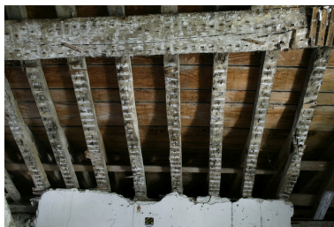
Charpente, détail des traces du lattis. Phot. Denis Pillet IVR52_20074401020NUCA
