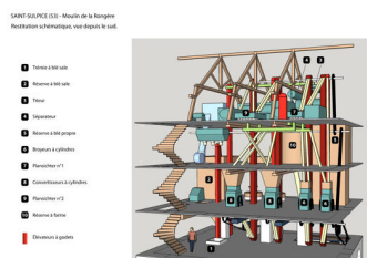
Vue axonométrique restituée de l'intérieur du moulin.
