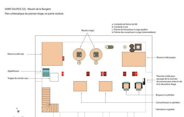
Plan schématique du premier étage.
