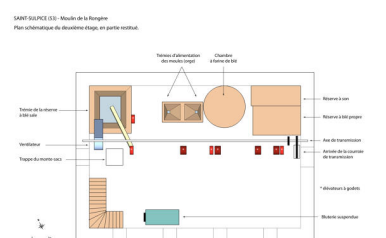
Plan schématique du deuxième étage.
