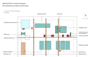
Plan schématique du comble.
