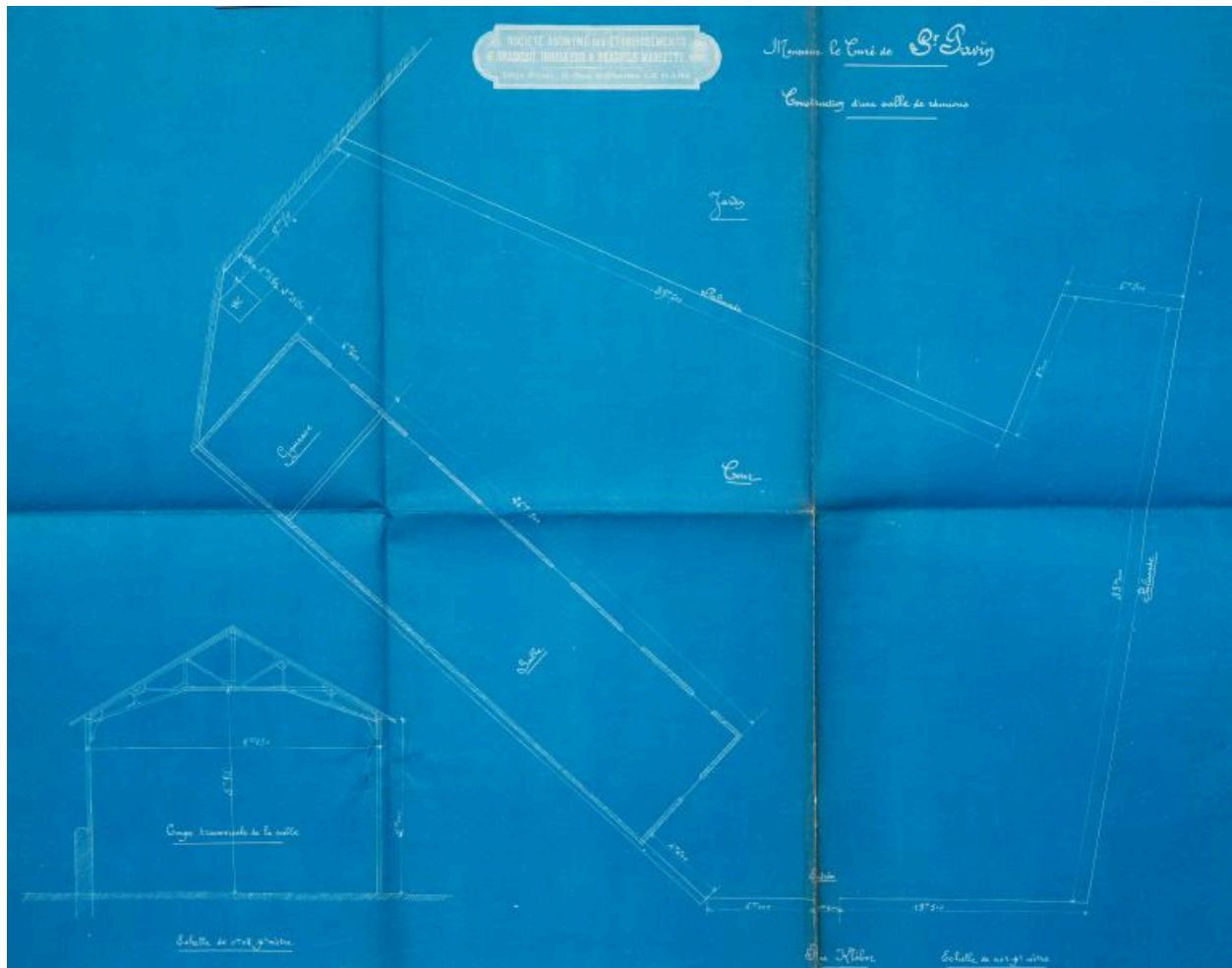
Plan de la salle dite "Kléber", 1908.
