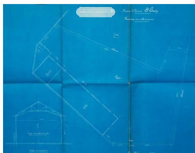
Plan de la salle dite "Kléber", 1908. Repro. Pierre-Bernard Fourny IVR52_20197201402NUCA
