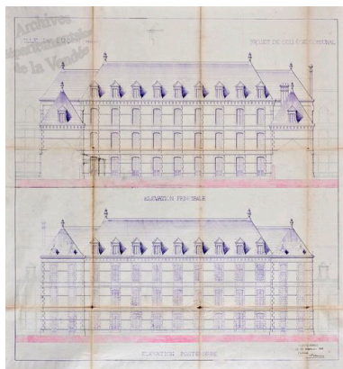
Projet simplifié par Arsène Charrier, le 25 septembre 1880 : élévations principale et postérieure (peu différentes du projet initial). Autr. Arsène Charrier, Phot. Patrice (reproduction) Giraud IVR52_20118500421NUCA
