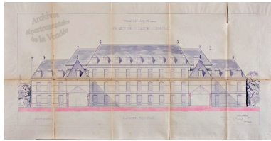
Projet initial par Arsène Charrier, le 25 juillet 1880 : élévation principale. Autr. Arsène Charrier, Phot. Patrice (reproduction) Giraud IVR52_20118500430NUCA
