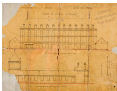
Projet définitif par Arsène Charier, le 20 décembre 1880 : élévation antérieure du bâtiment principal et élévation postérieure sur les classes. Autr. Arsène Charrier, Phot. Patrice (reproduction) Giraud IVR52_20118500427NUCA
