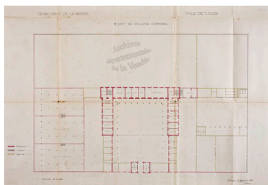
Deuxième modification par Arsène Charrier, le 23 novembre 1880 : plan d'ensemble. Autr. Arsène Charrier, Phot. Patrice (reproduction) Giraud IVR52_20118500424NUCA
