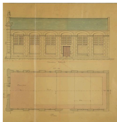
Plan et élévation latérale du gymnase par Bordelais, en 1899. Autr. Emile II Bordelais, Phot. Patrice (reproduction) Giraud IVR52_20068500156NUCA
