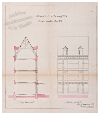
Première modification par Arsène Charrier, le 6 novembre 1880 : coupe et élévation partielle. Autr. Arsène Charrier, Phot. Patrice (reproduction) Giraud IVR52_20118500423NUCA
