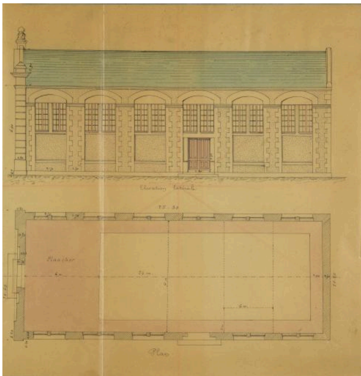
Plan et élévation latérale du gymnase par Bordelais, en 1899.
