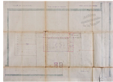
Projet simplifié par Arsène Charrier, le 25 septembre 1880 : plan d'ensemble (simplifié par rapport au projet initial). Autr. Arsène Charrier, Phot. Patrice (reproduction) Giraud IVR52_20118500420NUCA
