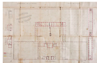
Autre modification par Arsène Charrier, le 17 novembre 1880 : plan général. Autr. Arsène Charrier, Phot. Patrice (reproduction) Giraud IVR52_20118500422NUCA
