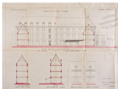
Deuxième modification par Arsène Charrier, le 23 novembre 1880 : élévation principale et coupes. Autr. Arsène Charrier, Phot. Patrice (reproduction) Giraud IVR52_20118500425NUCA
