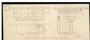
Plans des écuries donnant place de la Brianderie. Phot. Patrick (reproduction) Jean IVR52_20134401174NUCA
