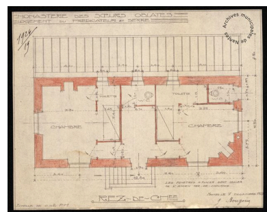
Plan de la maison du prédicateur et des serres.
