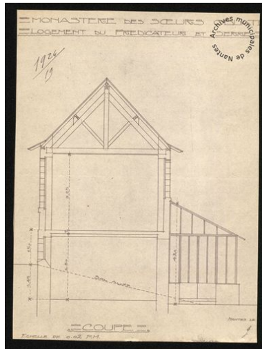
Coupe de la maison du prédicateur et des serres. Phot. Patrick (reproduction) Jean IVR52_20134401176NUCA
