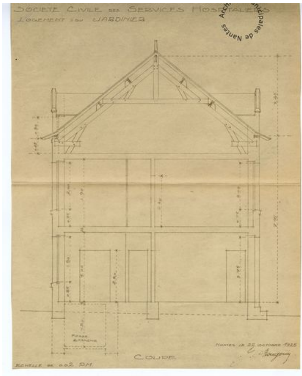
Coupe de la maison du jardinier.
