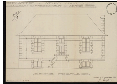
Elévation de la maison du prédicateur et des serres Phot. Patrick (reproduction) Jean IVR52_20134401172NUCA
