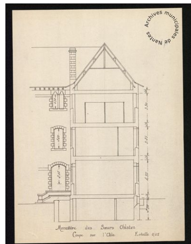
Coupe de la maison mère. Phot. Patrick (reproduction) Jean IVR52_20134401169NUCA
