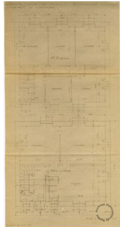
Plan de la maison du jardinier. Phot. Patrick (reproduction) Jean IVR52_20134401180NUCA
