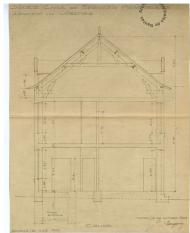
Coupe de la maison du jardinier. Phot. Patrick (reproduction) Jean IVR52_20134401181NUCA
