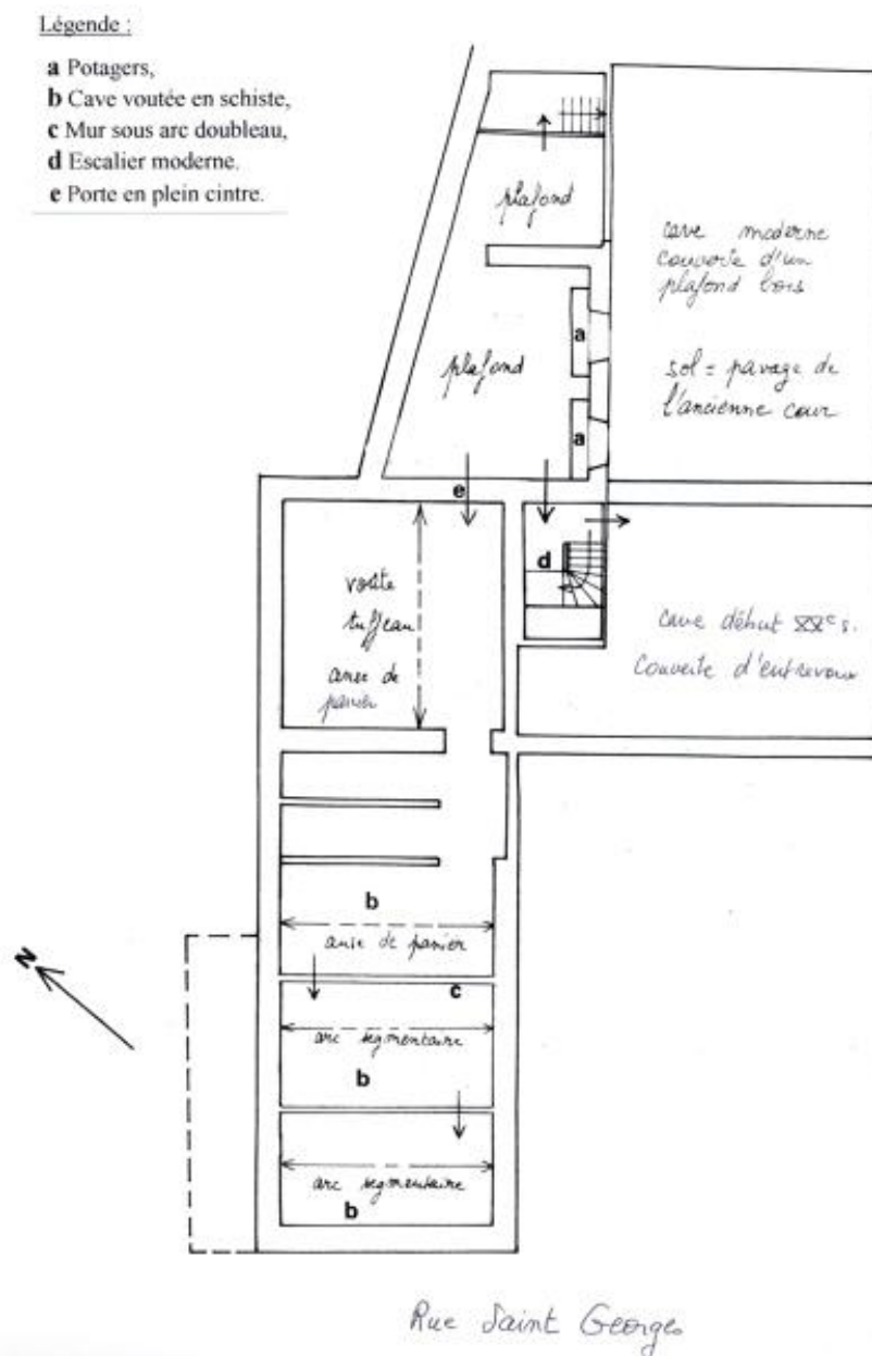
Plan schématique du niveau de cave.
