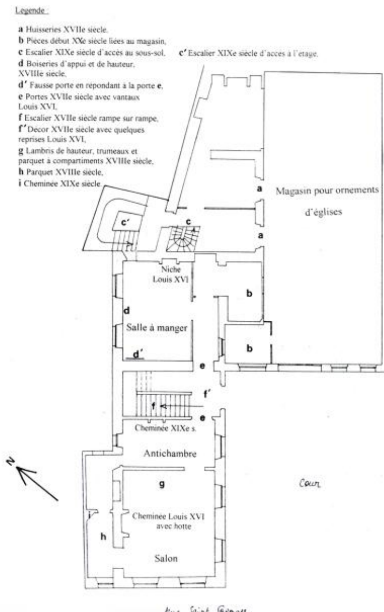
Plan du rez-de-chaussée, d'après le plan dessiné par M. Briand le 07/01/1967 à Angers (AP).
