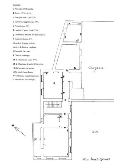
Plan du premier étage, d'après le plan dessiné par M. Briand le 07/01/1967 à Angers (AP).
