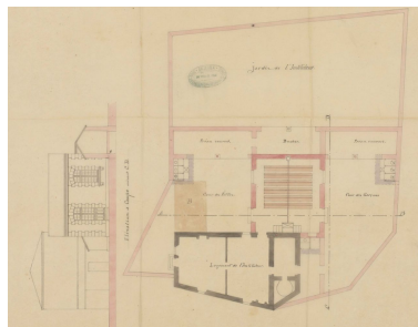
Projet de construction d'une salle de classe à Aziré, par Arsène Charrier, 10 janvier 1878 : plan et élévation nord. Repro. Yannis Suire IVR52_20238502274NUCA
