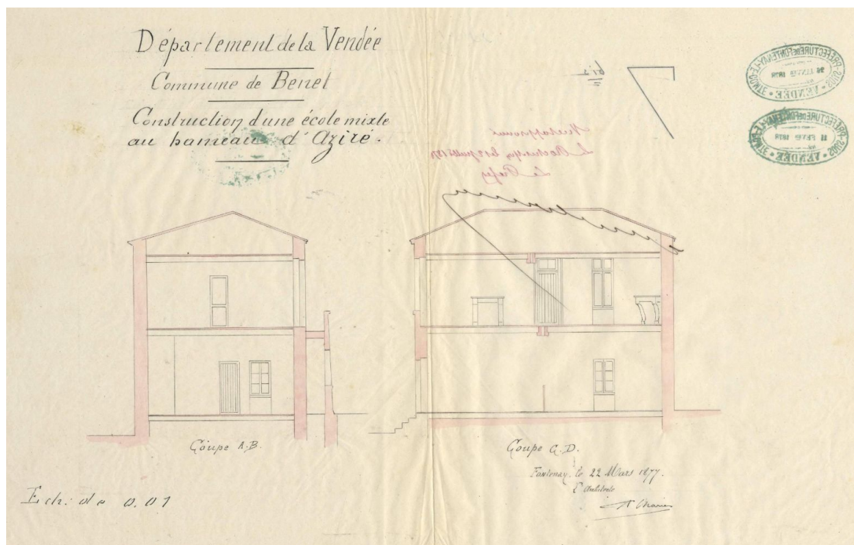
Projet d'aménagement d'une école à Aziré, par Arsène Charrier, 22 mars 1877 : coupes de la maison.
