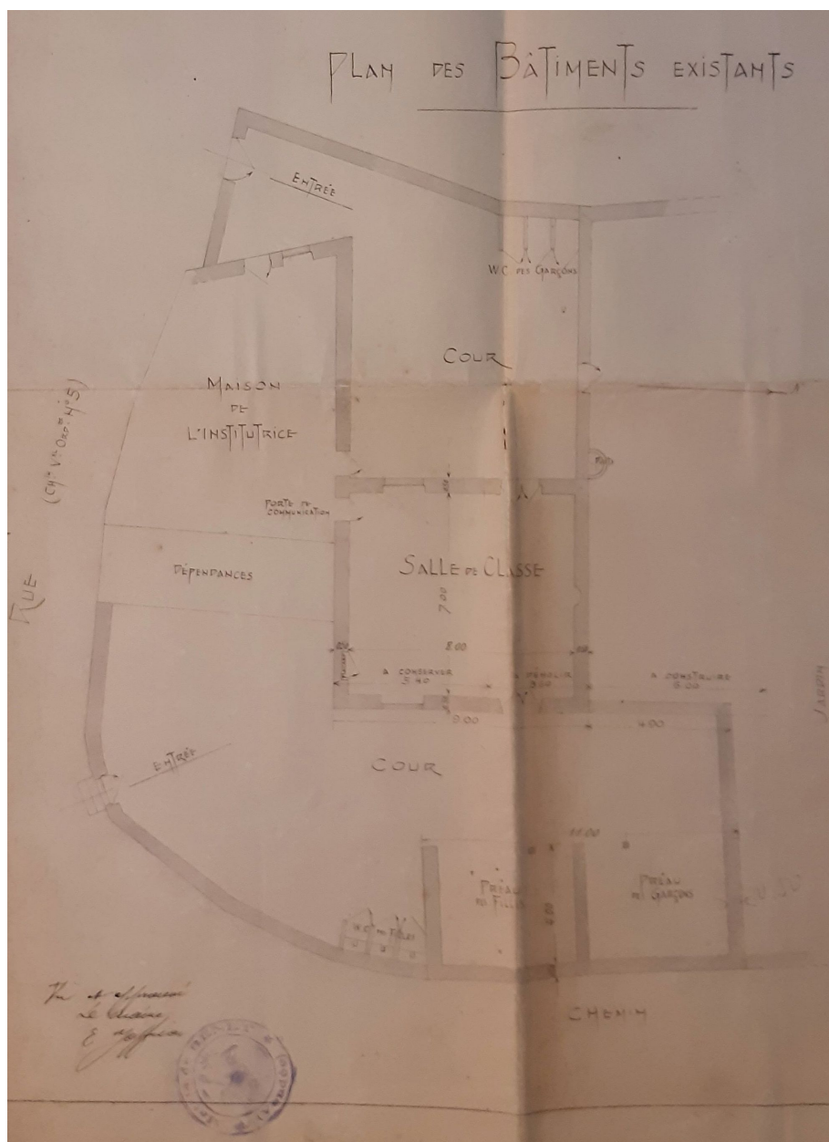
Plan de l'école avant agrandissement de la salle de classe, par Ariste Fourier, 31 mai 1928.
