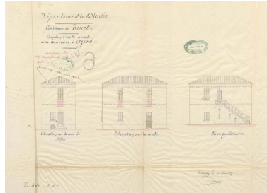
Projet d'aménagement d'une école à Aziré, par Arsène Charrier, 22 mars 1877 : élévations de la maison. Repro. Yannis Suire IVR52_20238502275NUCA
