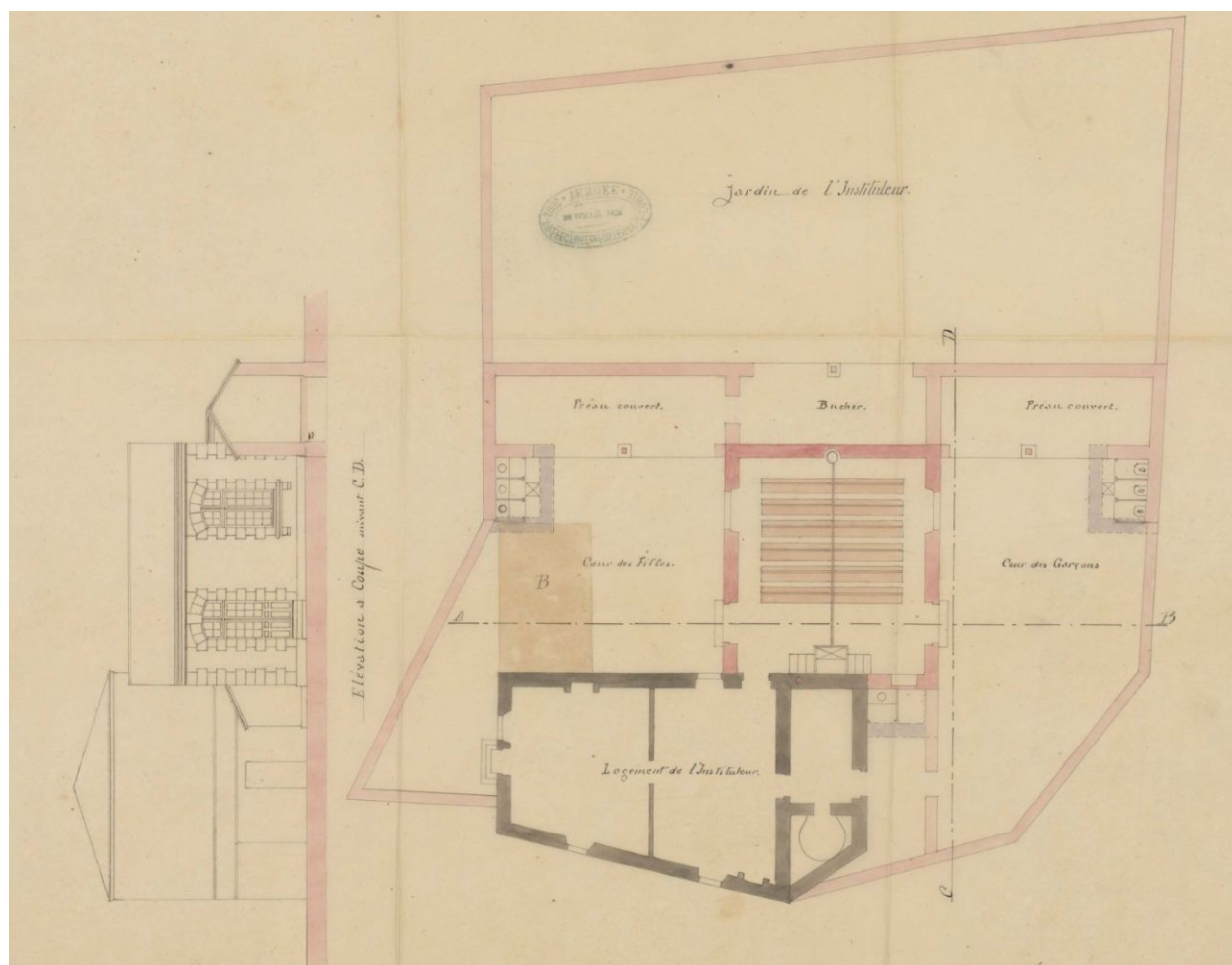
Projet de construction d'une salle de classe à Aziré, par Arsène Charrier, 10 janvier 1878 : plan et élévation nord.
