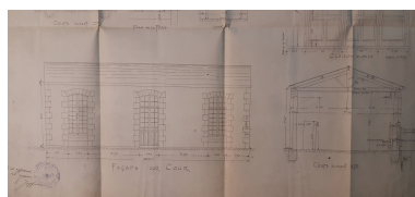
Projet d'agrandissement de la salle de classe, par Ariste Fourier, 31 mai 1928 : coupe et élévation nord. Repro. Yannis Suire IVR52_20238502305NUCA
