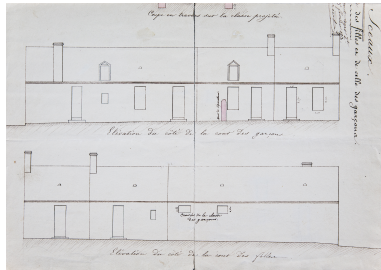
Des plans de l'ancienne école, rue Saint-Eloi, 1850. Repro. Pierre-Bernard Fourny IVR52_20187202621NUCA
