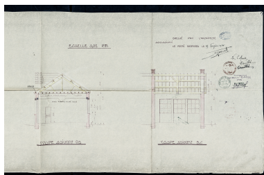
Des plans de construction d'une classe, 1931. Repro. Pierre-Bernard Fourny, Autr. Marcel Jacquet IVR52_20197200142NUCA
