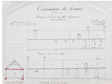
Des plans de l'ancienne école, rue Saint-Eloi, 1855. Repro. Pierre-Bernard Fourny IVR52_20187202619NUCA
