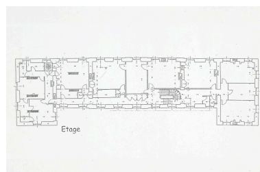
Plan de l'étage, par M. Banchereau. Autr. Banchereau, Repro. François Lasa IVR52_20065300816NUCA
