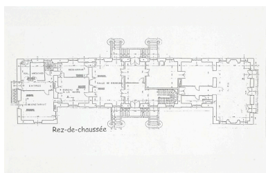
Plan du rez-de-chaussée, avec la fonction des pièces occupées par la mairie, par M. Banchereau. Autr. Banchereau, Repro. François Lasa IVR52_20065300815NUCA
