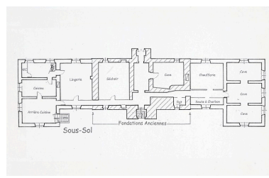
Plan du sous-sol, avec la fonction des pièces avant la transformation en mairie, par L. Avila. Autr. Laëtitia Avila, Repro. François Lasa IVR52_20065300818NUCA
