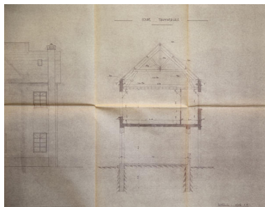
Elévation et coupe pour l'agrandissement de l'école Garnier Pagès, 1937. Repro. Pierre-Bernard Fourny IVR52_20197202907NUCA
