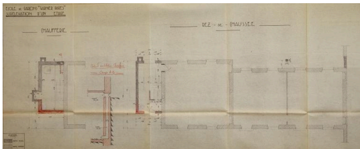
Plan de l'étage projeté à l'école Garnier Pagès, 1937.
