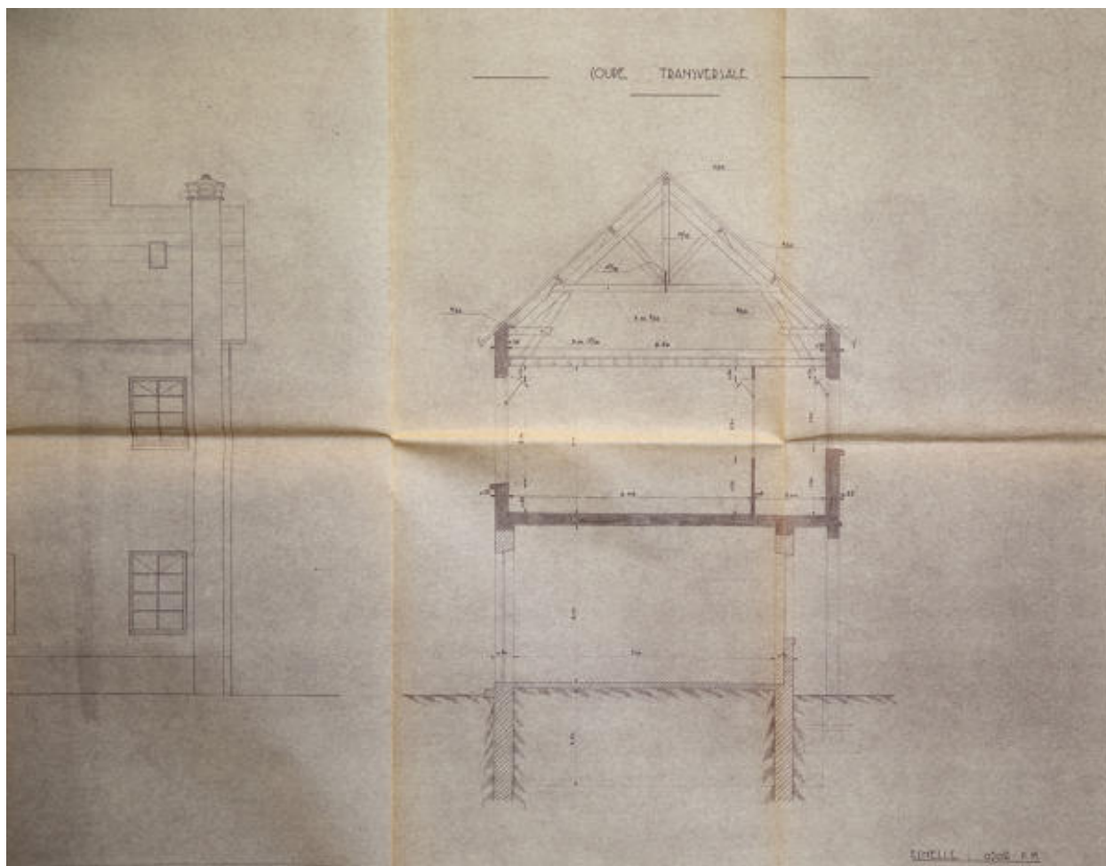
Elévation et coupe pour l'agrandissement de l'école Garnier Pagès, 1937.
