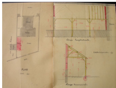
La Maison d'école de garçons, détail : construction d'un préau dans la cour antérieure. Phot. Christine (reproduction) Toulhier IVR52_20057203894NUCA
