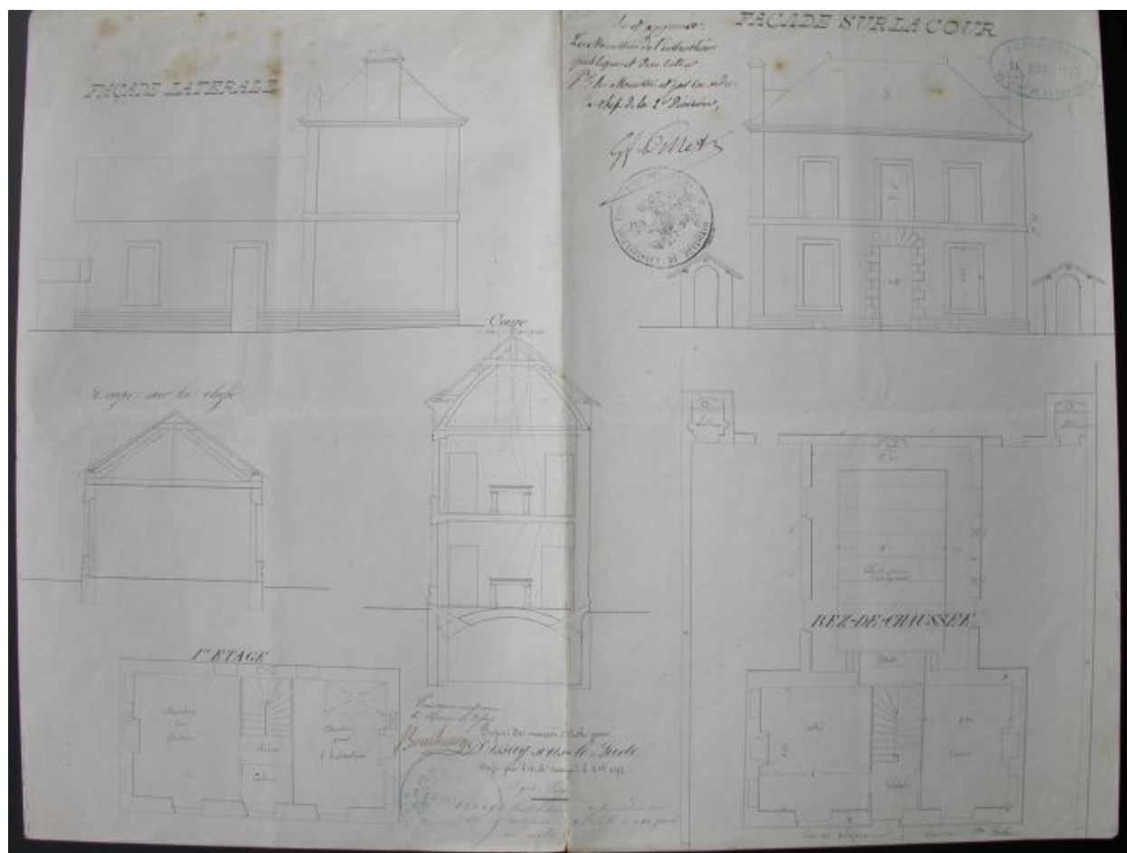
Plan, coupe et élévation de la Maison d'école.
