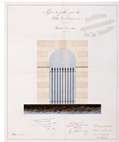
Projet de grille pour les halles, élévation d'une travée. Dessin de A. Buquet, architecte et inspecteur diocésain, le 16 mai 1859. Autr. A. Buquet, Phot. Patrice (reproduction) Giraud IVR52_20118500384NUCA
