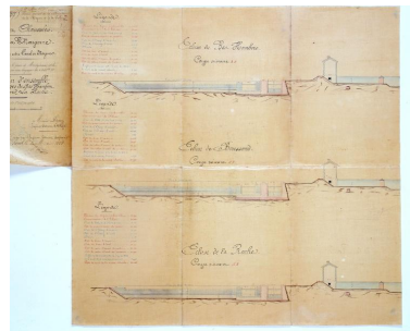
Projet de canalisation de la Mayenne entre le Bas-Hambert et Grenoux : coupes longitudinales des barrages de Bas-Hambert, Boussard et la Roche. Autr. Charles Dupuy, Repro. François Lasa IVR52_20025300135XA
