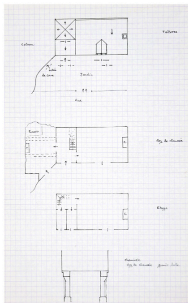
Plan schématique (toitures, RdC, 1er étage) et croquis de la cheminée, établis lors du pré-inventaire de 1979 (nord droite).
