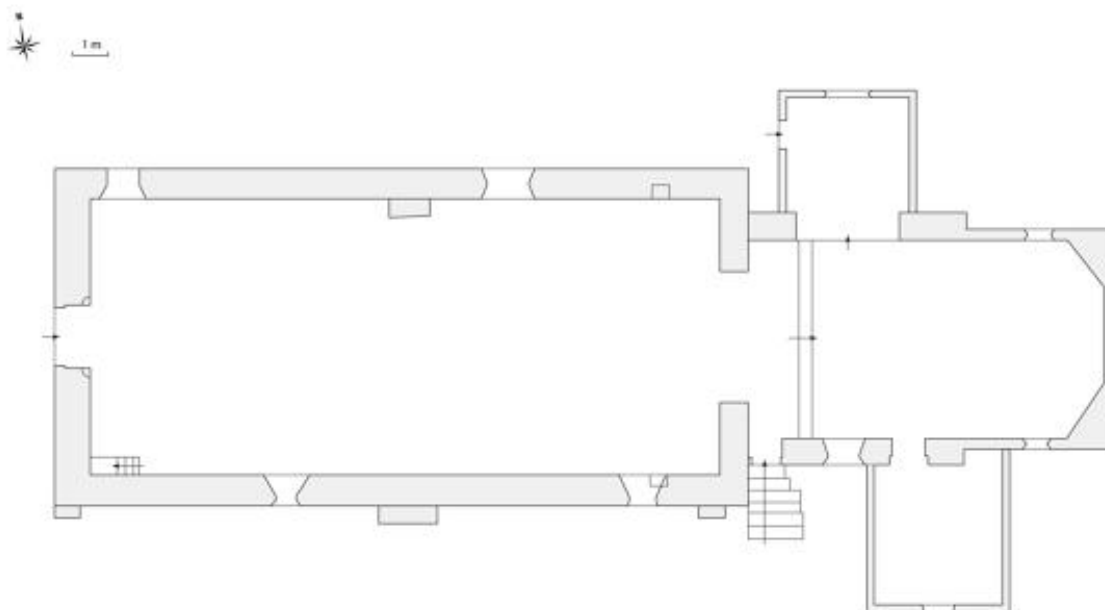
Lavenay (72) - Église paroissiale Plan schématique Relevé - V. Desvigne - mai 2015
