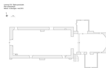
Plan de l'église paroissiale, Virginie Desvigne, Région Pays de la Loire, 2015. Dess. Virginie Desvigne IVR52_20157201457NUDA
