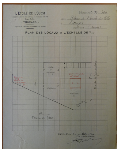
Plan à l'appui de la demande d'autorisation de création d'un débit de pétroles, 20 juillet 1934. Phot. Yannis (reproduction) Suire IVR52_20228501062NUCA
