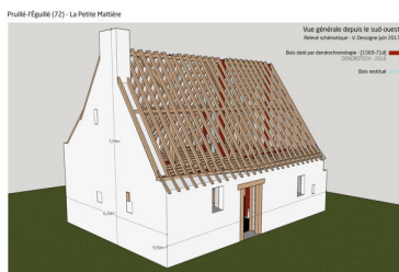
Relevé schématique de la maison vue depuis le sud-ouest, V. Desvigne, 2017. Dess. Virginie Desvigne IVR52_20187202636NUDA
