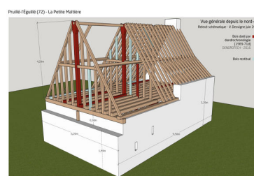
Relev  sch matique de la maison vue depuis le nord-est, V. Desvigne, 2017. Dess. Virginie Desvigne IVR52_20187202638NUCA
