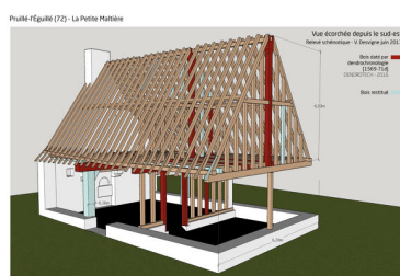
Vue  corch e de la maison depuis le sud-est, V. Desvigne, 2017. Dess. Virginie Desvigne IVR52_20187202637NUCA
