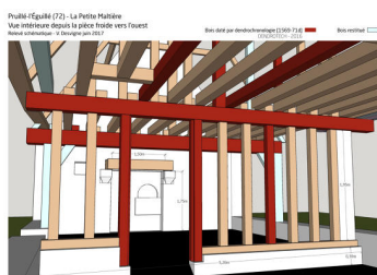
Relev  sch matique : vue int rieure depuis la pi ce froide vers l'ouest, V. Desvigne, 2017. Dess. Virginie Desvigne IVR52_20187202639NUCA
