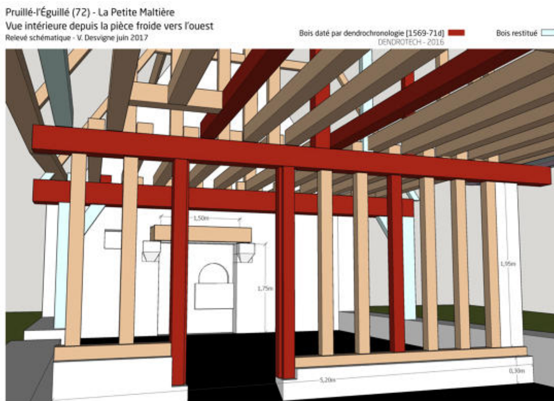
Relevé schématique : vue intérieure depuis la pièce froide vers l'ouest, V. Desvigne, 2017.
