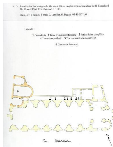
Localisation des vestiges du onzième siècle (?) sur un plan repris d'un relevé de H. Enguehard du 16 avril 1965. Ech. originale 1 : 100. Dess. I. Frager IVR52_20034901031A4
