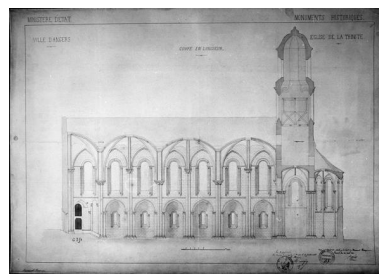
Coupe longitudinale, par Ch. Joly-Leterme, 1862. Repro. François Lasa IVR52_19934902987X
