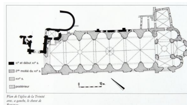
Plan de l'église et de sa sacristie avec, à gauche, le choeur et le croisillon sud de l'abbaye du Ronceray, par Yves Blomme. Repro. François Lasa IVR52_20054901371NUCA
