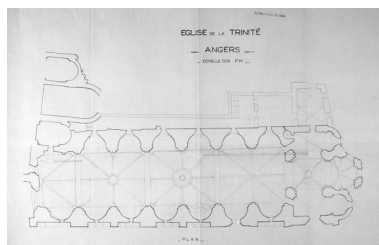
Plan, par Bernard Vitry, 1950. Repro. François Lasa IVR52_19934902989X
