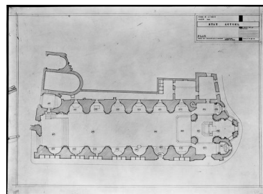
Plan au sol de l'église paroissiale de la Trinité, par H. Enguehard, 1965. Repro. François Lasa IVR52_19794903254P
