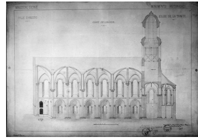
Coupe longitudinale, par Ch. Joly-Leterme, 1862. Repro. François Lasa IVR52_19934902987X
