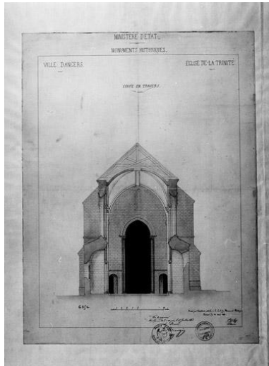
Nef, septième travée : coupe transversale vers l'est, par Charles Joly-Leterme, 1862. Repro. François Lasa IVR52_19934902985X
