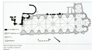
Plan de l'église et de sa sacristie avec, à gauche, le chœur et le croisillon sud de l'abbaye du Ronceray, par Yves Blomme. Repro. François Lasa IVR52_20054901371NUCA
