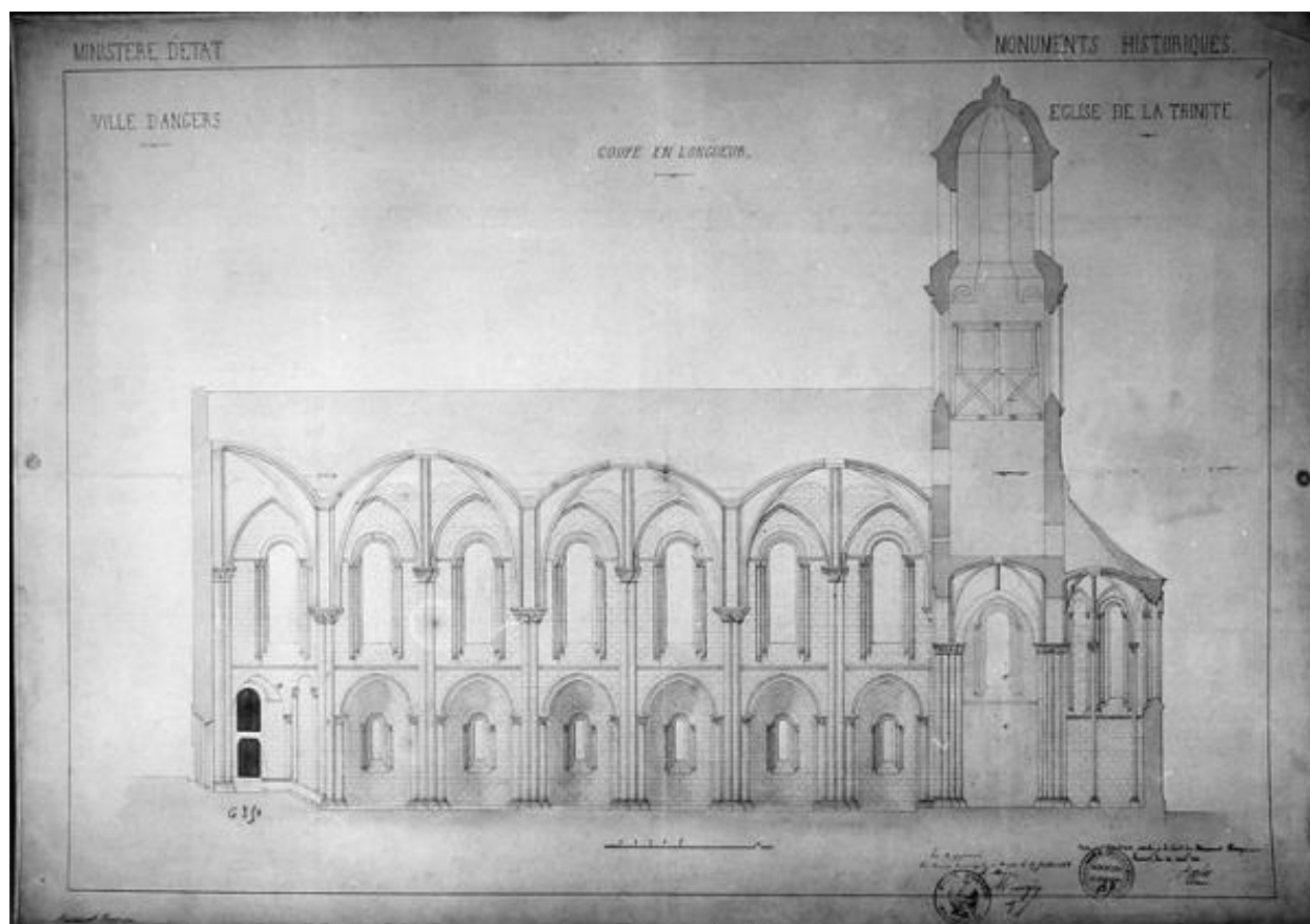
Coupe longitudinale, par Ch. Joly-Leterme, 1862.
