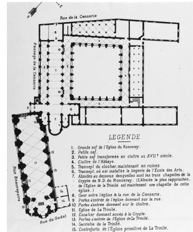
Plan au sol, [v. 1895]. Repro. Patrice Giraud IVR52_20044905600NUC
