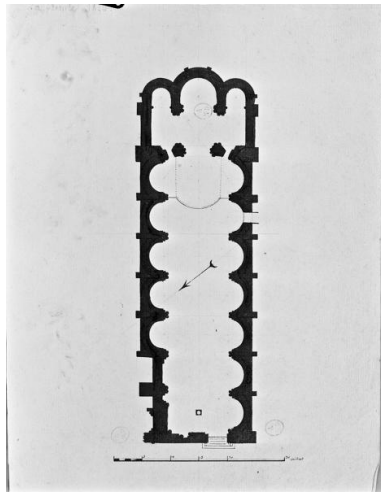
Plan de 1826 de la Trinité. Repro. Patrice Giraud IVR52_19774900870X
