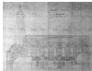
Elévation latérale nord, dessin, par B. Vitry, 1950. Repro. François Lasa IVR52_19934902983X
