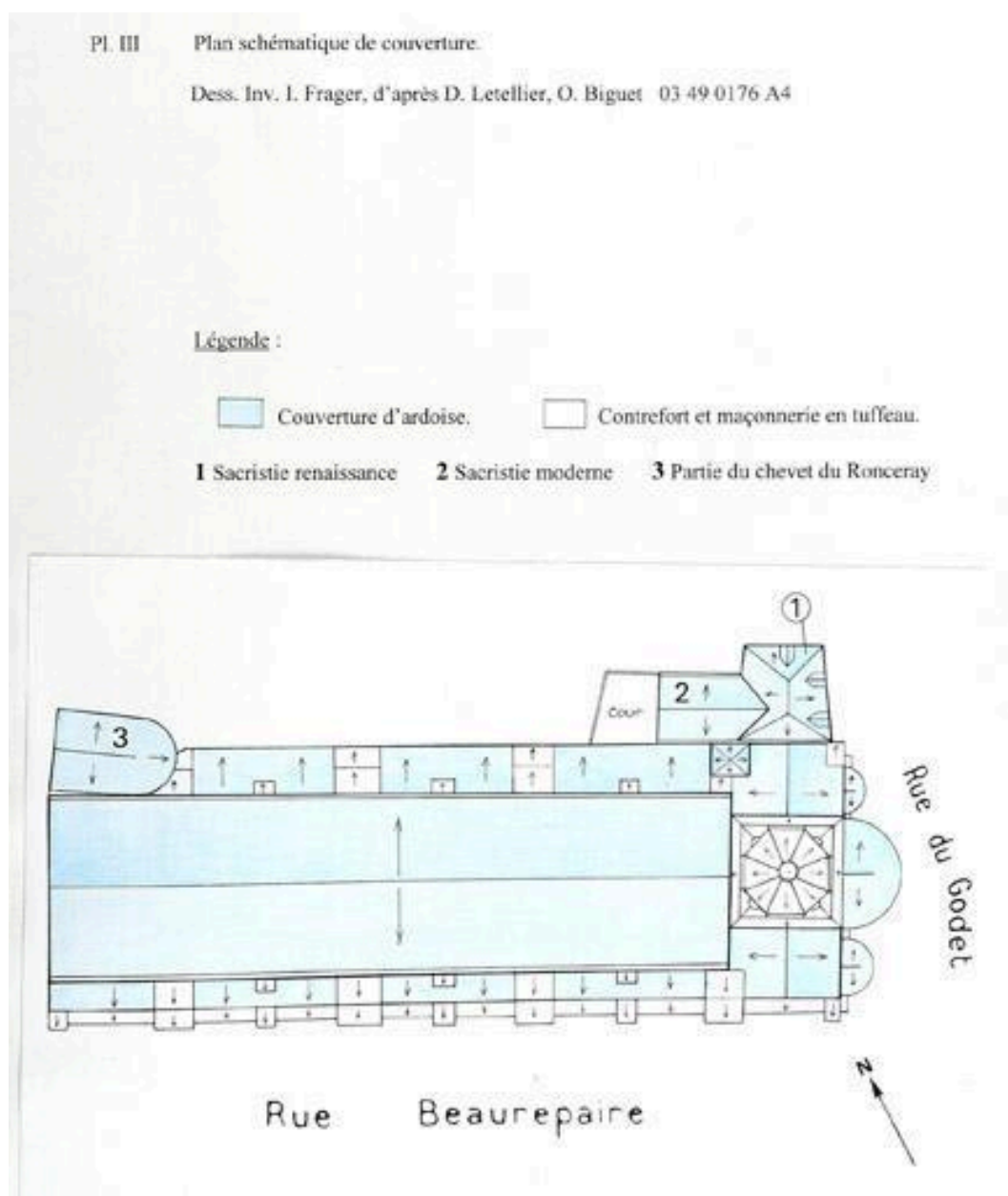
Plan schématique de couverture.
