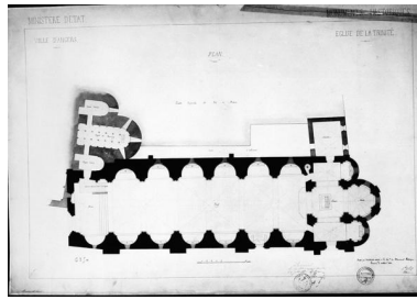
Plan, par Ch. Joly-Leterme, 1862. Repro. François Lasa IVR52_19934902986X
