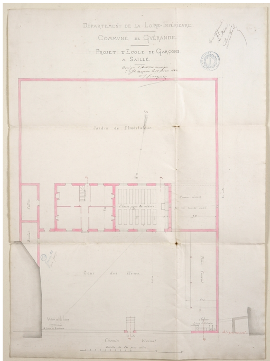
Projet d'école de garçons à Saillé, dressé par A. Pinguet (1882). Plan au sol.
