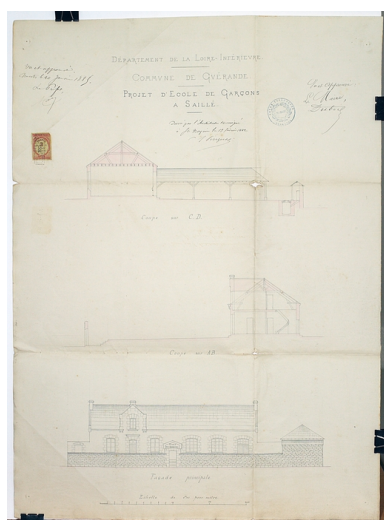
Projet d'école de garçons à Saillé, dressé par A. Pinguet (1882). Coupes et élévation. Phot. Denis (reproduction) Pillet IVR52_20084401550NUCA
