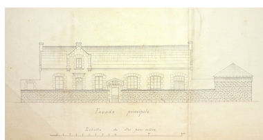
Projet d'école de garçons à Saillé, dressé par A. Pinguet (1882). Détail. Élévation de la façade principale. Phot. Denis (reproduction) Pillet IVR52_20084401553NUCA
