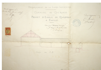
Projet d'école de garçons à Saillé, dressé par A. Pinguet (1882). Détail. Coupe est-ouest. Phot. Denis (reproduction) Pillet IVR52_20084401551NUCA
