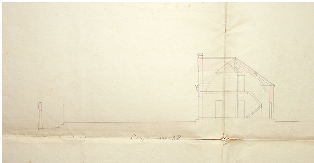
Projet d'école de garçons à Saillé, dressé par A. Pinguet (1882). Détail. Coupe nord-sud.
