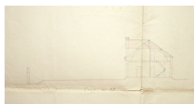
Projet d'école de garçons à Saillé, dressé par A. Pinguet (1882). Détail. Coupe nord-sud. Phot. Denis (reproduction) Pillet IVR52_20084401552NUCA
