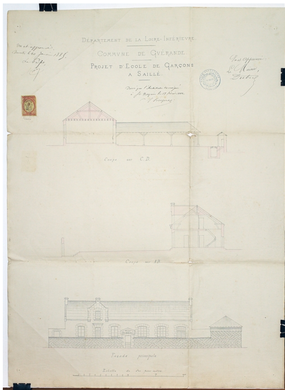
Projet d'école de garçons à Saillé, dressé par A. Pinguet (1882). Coupes et élévation.
