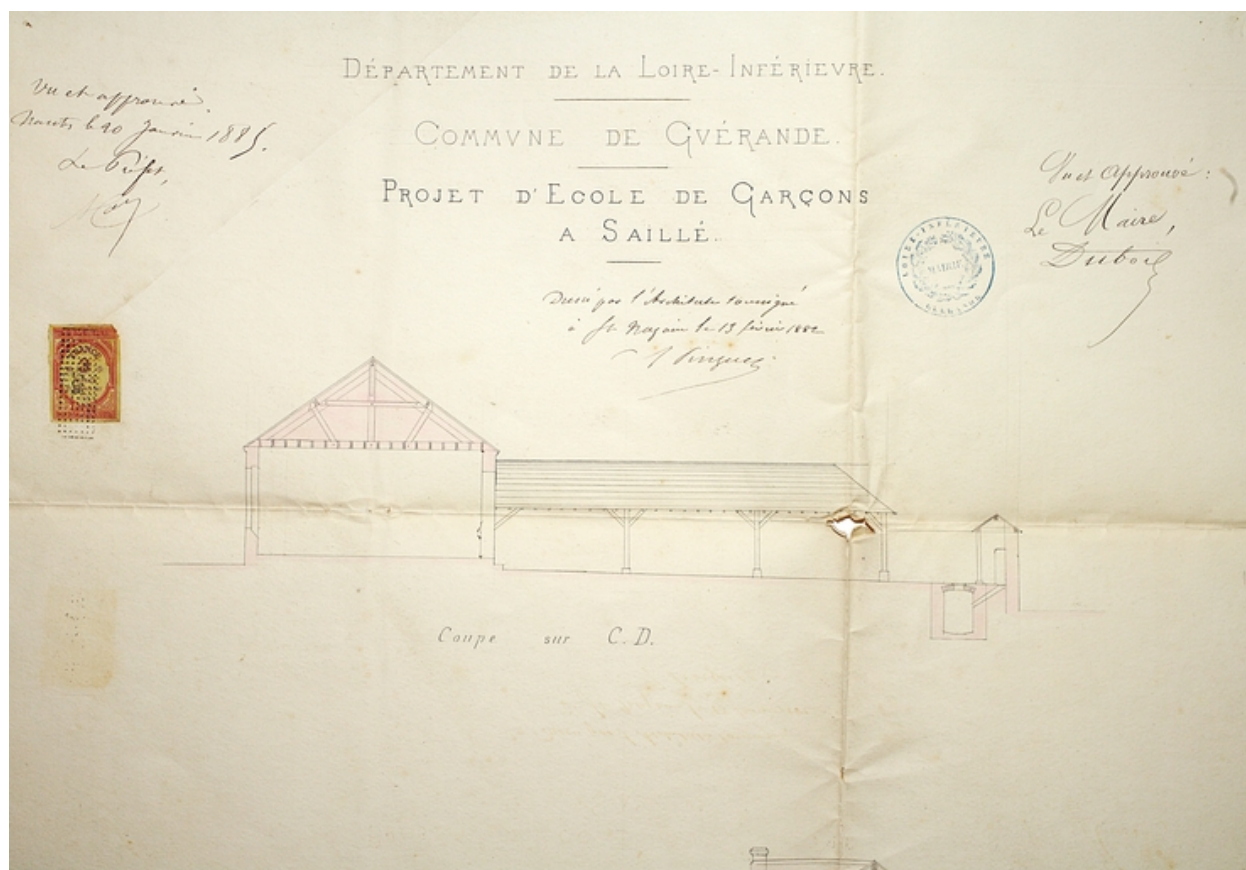
Projet d'école de garçons à Saillé, dressé par A. Pinguet (1882). Détail. Coupe est-ouest.
