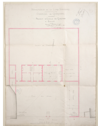
Projet d'école de garçons à Saillé, dressé par A. Pinguet (1882). Plan au sol. Phot. Denis (reproduction) Pillet IVR52_20084400417NUCA
