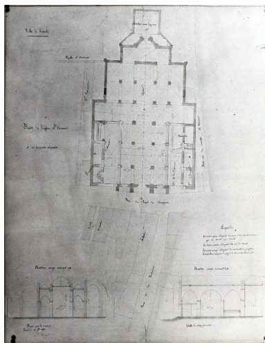
Projet d'agrandissement de l'église : plan, coupe transversale et coupe longitudinale. Autr. Eugène Boret, Phot. Patrice (reproduction) Giraud IVR52_19835300076X
