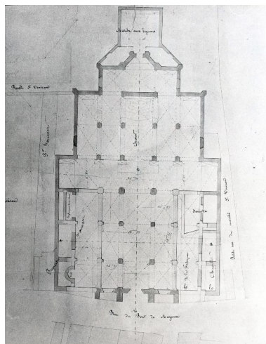
Projet d'agrandissement de l'église : plan projeté. Autr. Eugène Boret, Phot. Patrice (reproduction) Giraud IVR52_19835300077X
