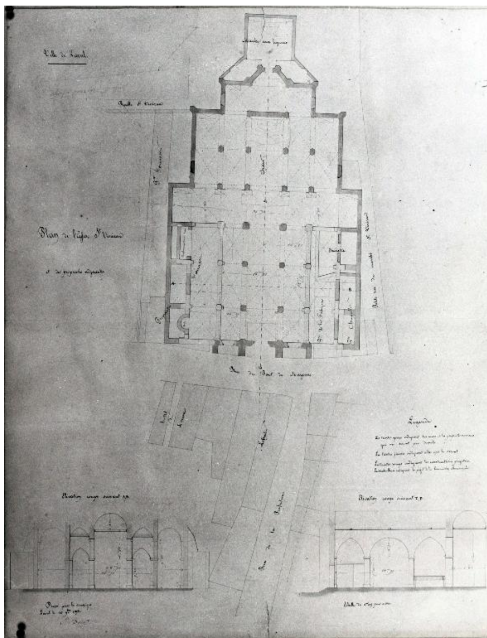
Projet d'agrandissement de l'église : plan, coupe transversale et coupe longitudinale.
