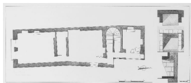
Plan du premier étage. Autr. Jocelyn Bourneuf, Phot. Denis (reproduction) Pillet IVR52_20044400663NUCA
