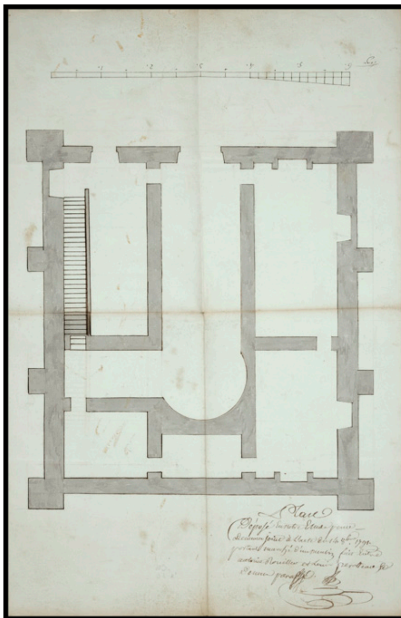
Plan du Moulin Perrotteau accompagnant le marché de construction passé le 14 octobre 1791.
