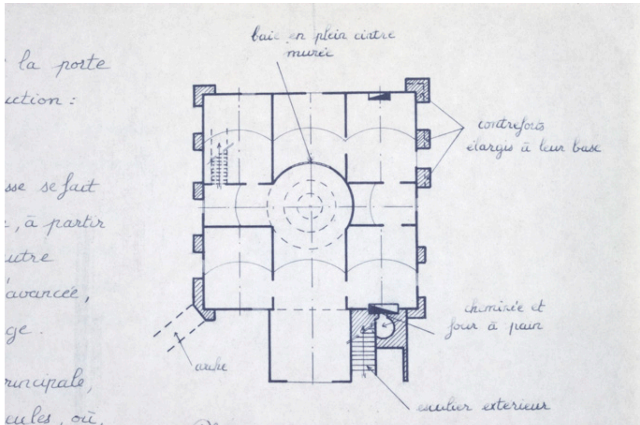
Plan schématique du Moulin Neuf, dressé en 1980.
