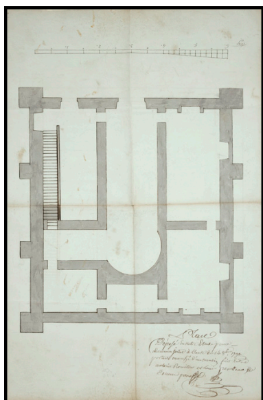
Plan du Moulin Perrotteau accompagnant le marché de construction passé le 14 octobre 1791. Autr. Antoine (?) Rouiller, Phot. Bruno Rousseau, Phot. Youenn (reproduction) Communeau IVR52_20114902015NUCA
