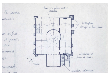
Plan schématique du Moulin Neuf, dressé en 1980. Phot. Bruno Rousseau, Phot. Youenn (reproduction) Communeau IVR52_20114902038NUCA
