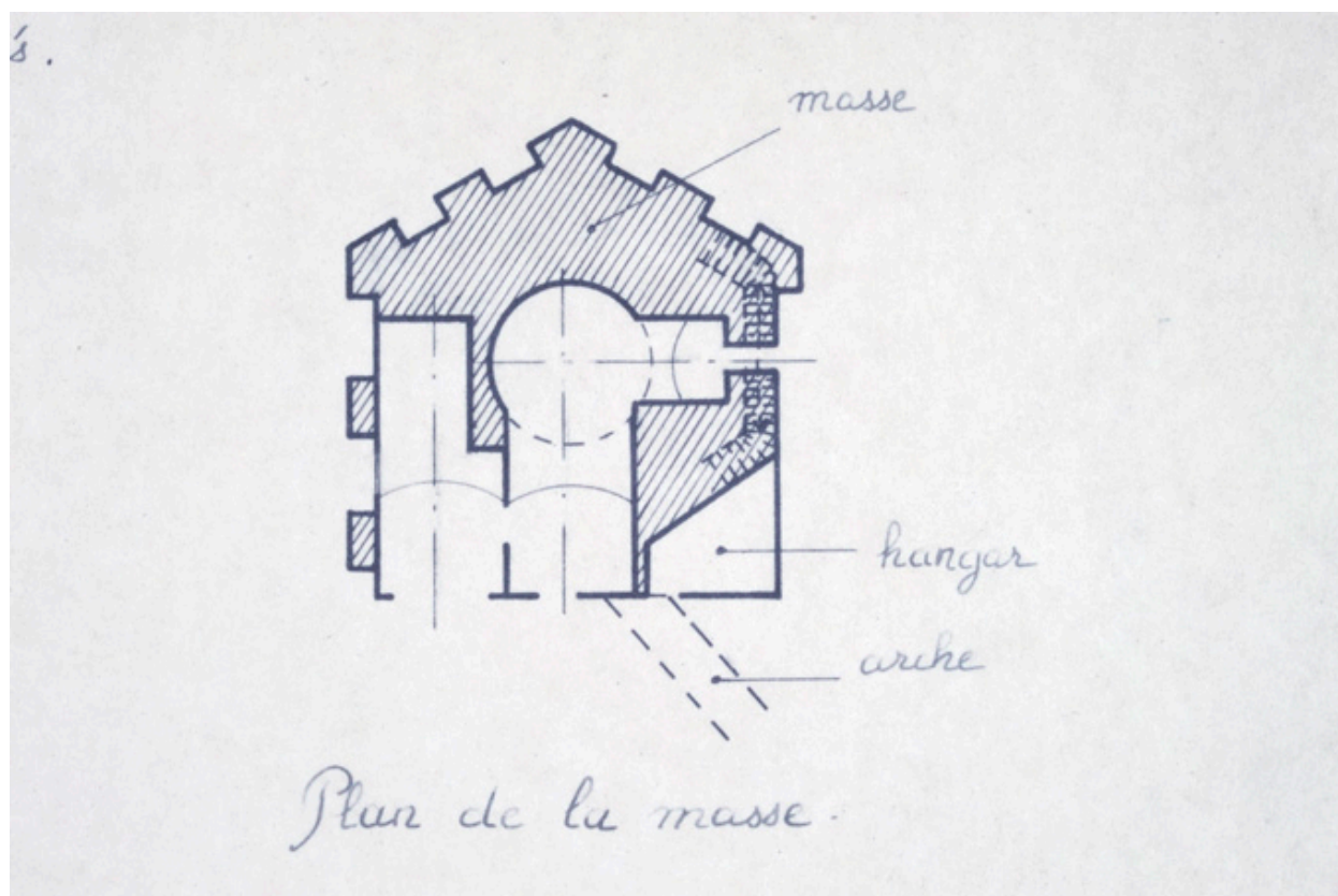
Plan schématique du moulin Picard, dressé en 1980.
