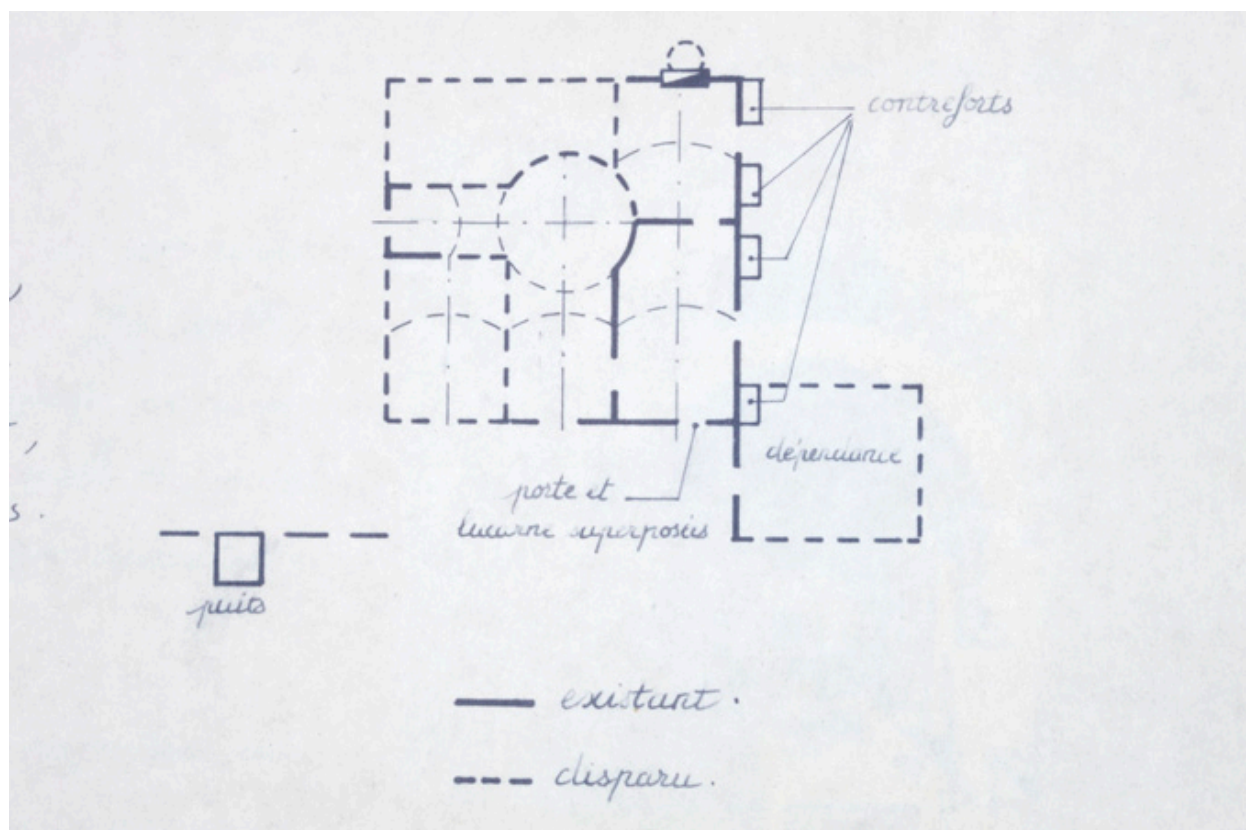
Plan schématique, dressé en 1980, du Moulin Bertrand (disparu).
