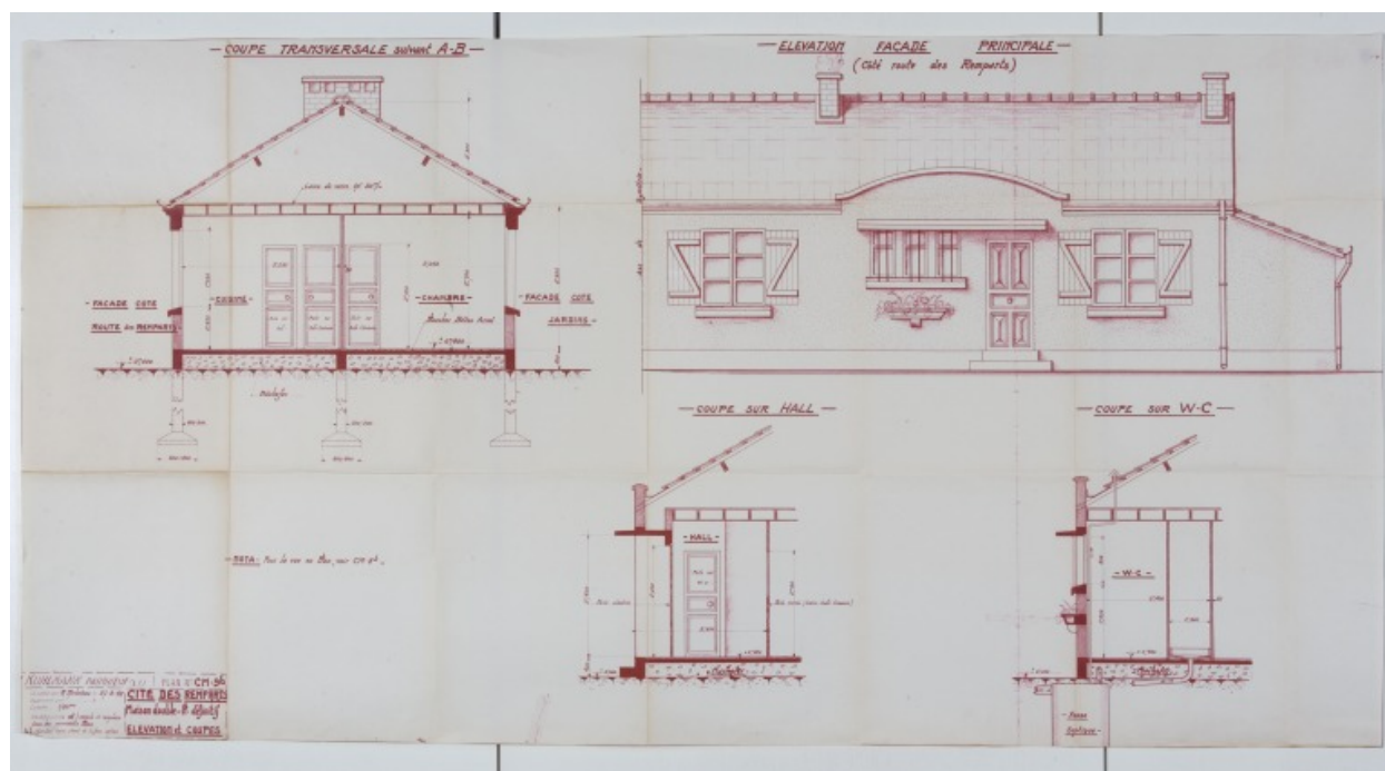
Elévation et coupe de la maison type, 1948.
