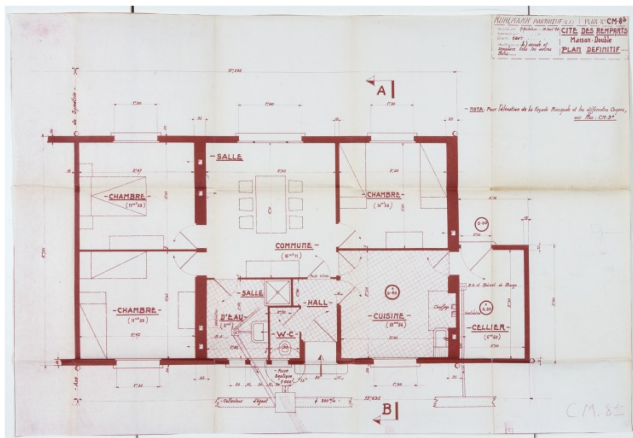
Plan d'une maison type, 1948.
