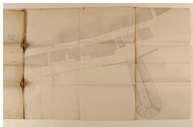
Plan des alignements à suivre pour les quais et cales de Paimboeuf, par Groleau, 1803, détail de la partie centrale. Autr. Mathurin Groleau, Phot. Frédéric (reproduction) Petot IVR52_20044400016NUCA
