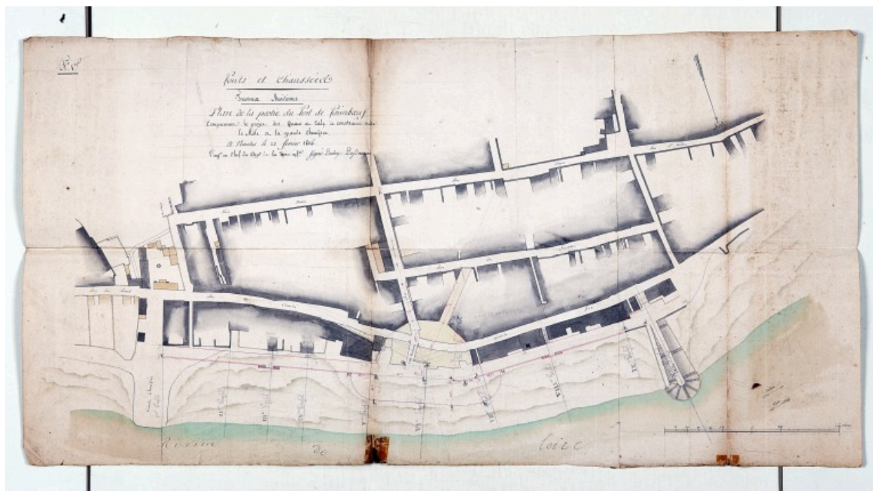
Projet des quais et cale à construire entre le nouveau môle et la cale située en amont dite la grande chaussée, par Duboys-Dessauzais, 1806.
