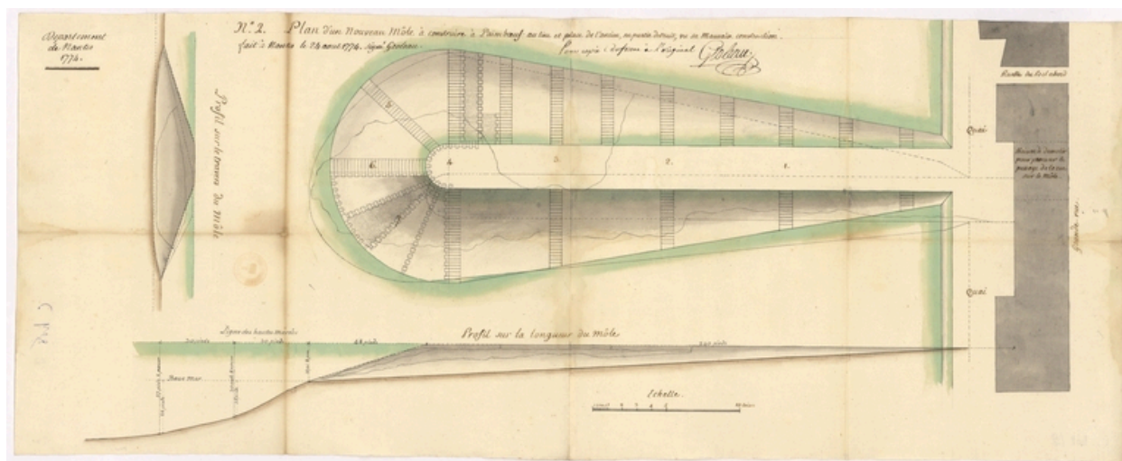
Plan du nouveau môle, par Groleau, 1774.
