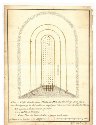
Plan, coupe, d'une partie du môle pour l'élever au-dessus des grandes marées, par Magin, 23 juillet 1767. Phot. Patrick (reproduction) Jean, Autr. Magin IVR52_20044400004NUCA
