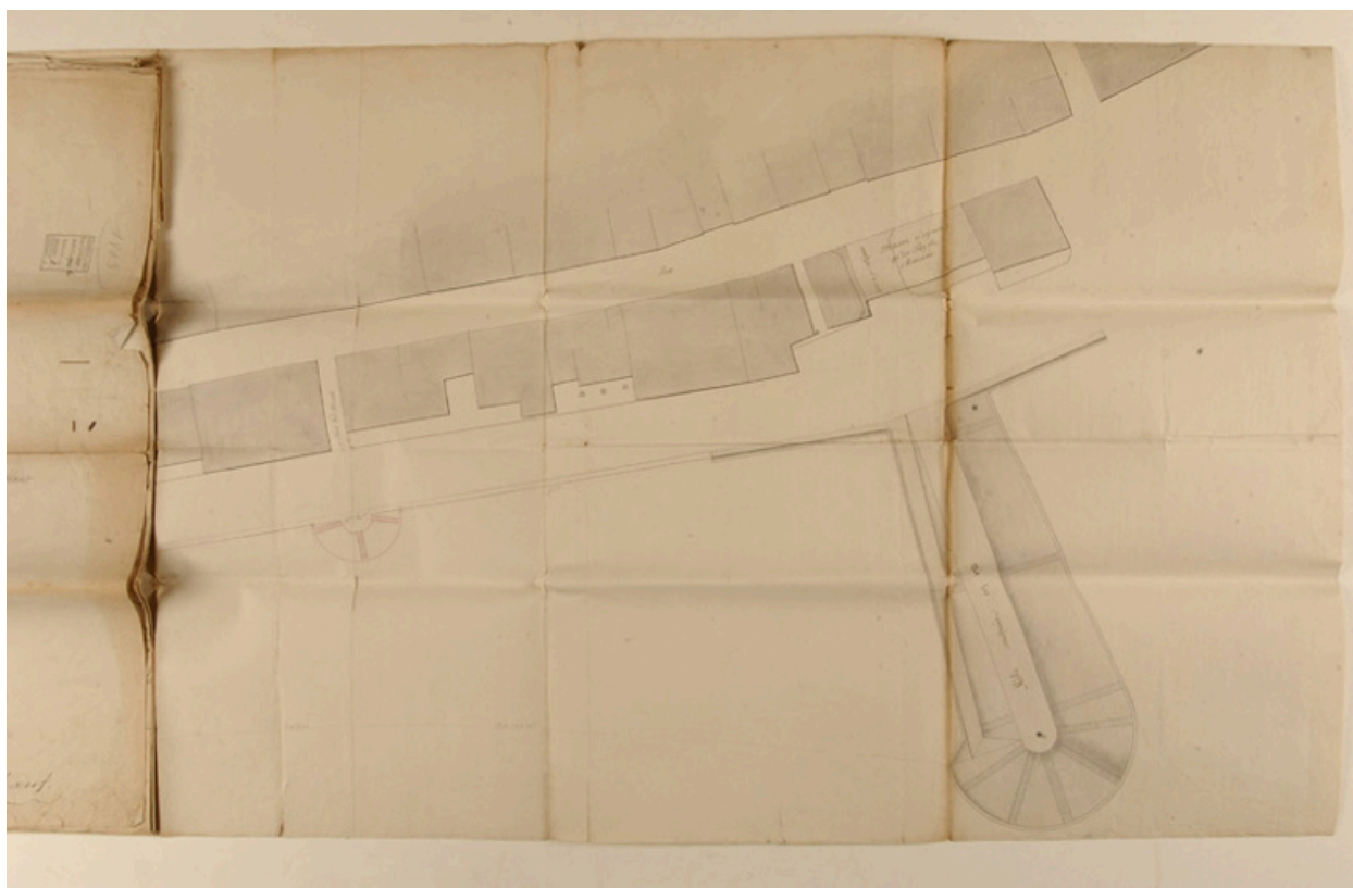
Plan des alignements à suivre pour les quais et cales de Paimboeuf, par Groleau, 1803, détail de la partie centrale.
