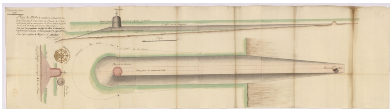
Plan du môle à construire vis à vis la Pierre à l'œil, par Groleau, 1776.
