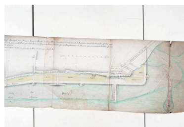
Plan d'une partie du port sur lequel figure le projet de deux nouveaux môles, par Groleau, 1778, détail de la partie aval. Autr. Mathurin Groleau, Phot. François Lasa IVR52_20054401236NUCA
