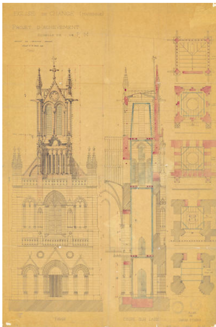
Les plans du clocher, par Garnier, 1890.
