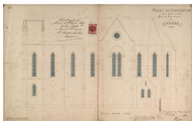
Le plan en élévation de la nef, du bras du transept sud et du chevet, par Renous, 1868. Repro. Allison Haugmard, Autr. Pierre-Aimé Renous IVR52_20215300215NUCA
