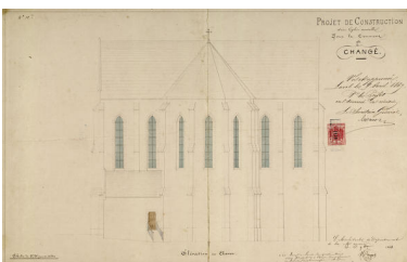
Le plan en élévation du chevet et des bras du transept, par Renous, 1868. Repro. Allison Haugmard, Autr. Pierre-Aimé Renous IVR52_20215300213NUCA
