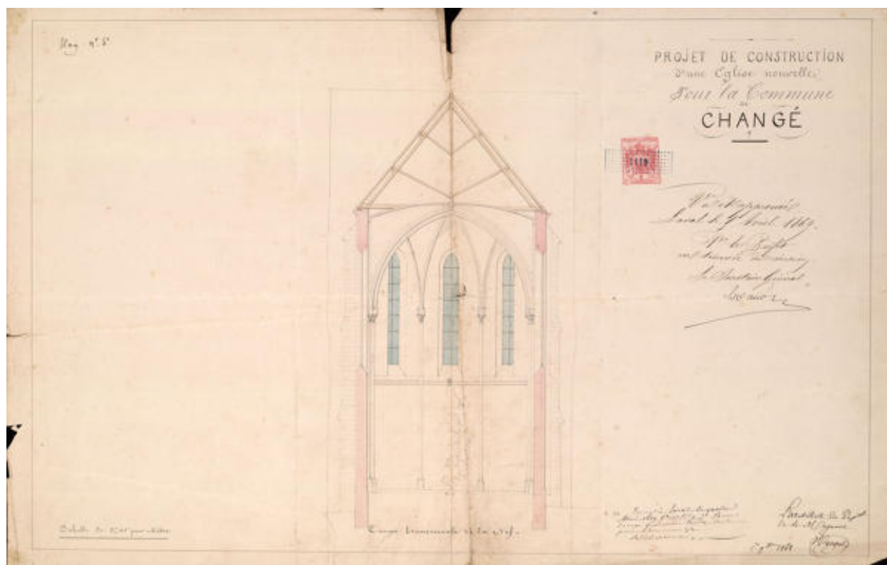
Le plan en élévation du chœur, par Renous, 1868.
