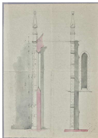
Les plans d'un contrefort, par l'architecte Louis Garnier, vers 1893. Repro. Allison Haugmard, Phot. Louis Garnier IVR52_20215301733NUCA
