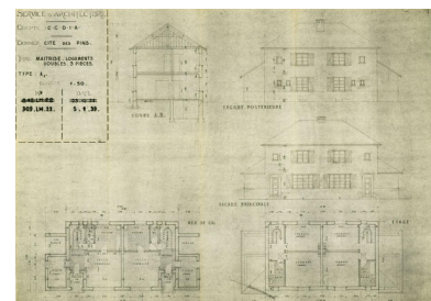
Plan, coupe et élévations des pavillons de maîtrise type A. IVR52_20217200109NUCA
