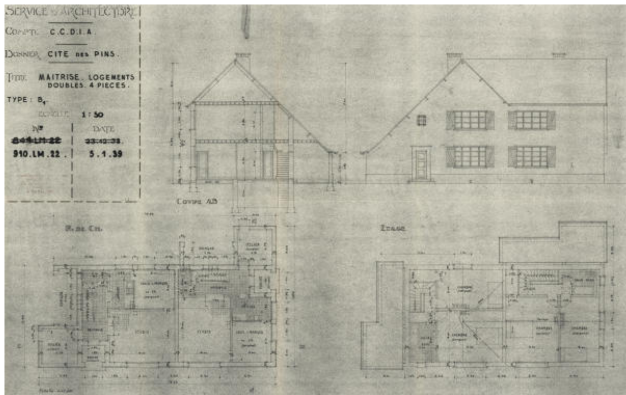
Plans, coupe et élévations des pavillons de maitrise de type B.
