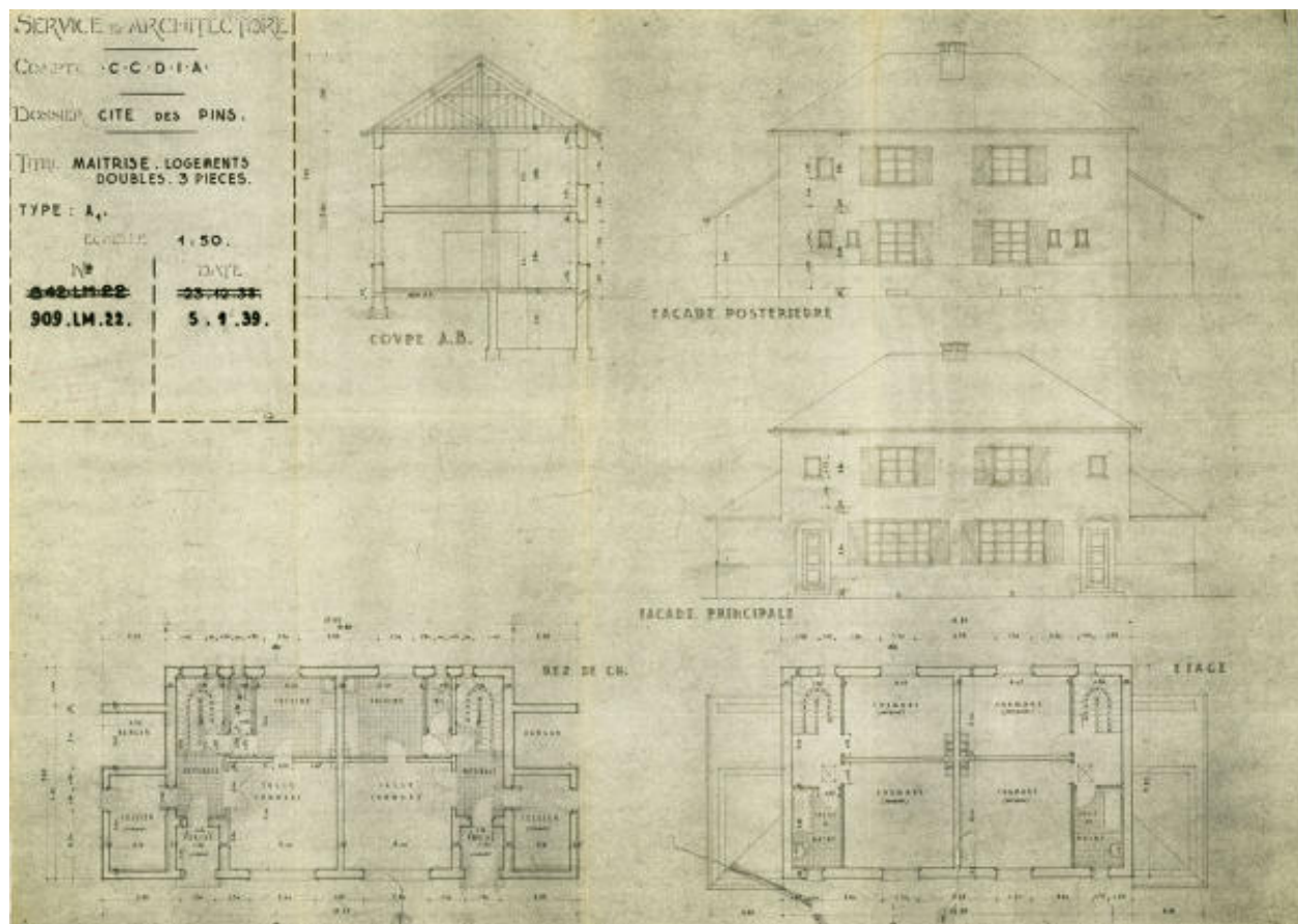
Plan, coupe et élévations des pavillons de maîtrise type A.
