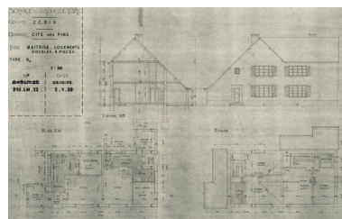
Plans, coupe et élévations des pavillons de maîtrise de type B. IVR52_20217200110NUCA
