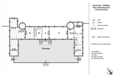
Plan schématique des rez- de-chaussée du logis. Dess. Julien Hardy IVR52_20087203089NUDA
