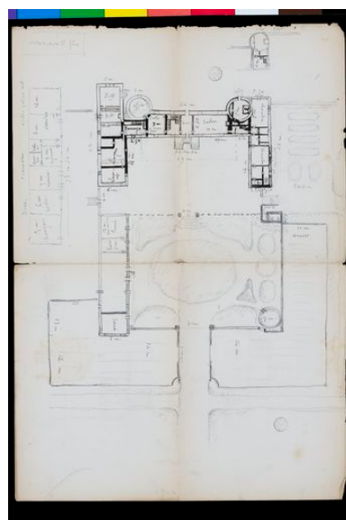
Plan schématique, 1ère moitié du XXe siècle ? Repro. François Lasa IVR52_20087201317NUCA
