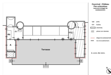
Plan schématique des sous-sol et étages de soubassement du logis. Dess. Julien Hardy IVR52_20087203088NUDA
