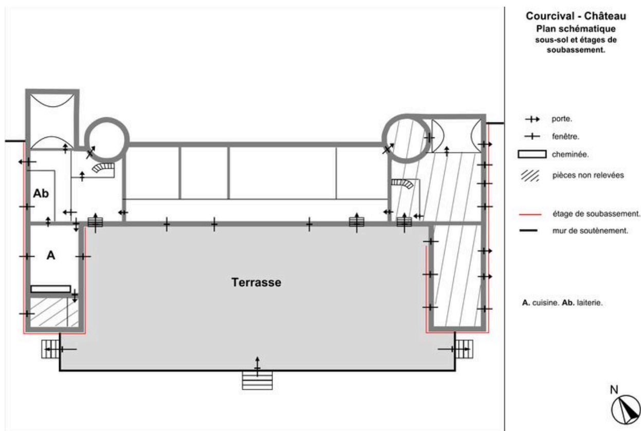
Plan schématique des sous-sol et étages de soubassement du logis.
