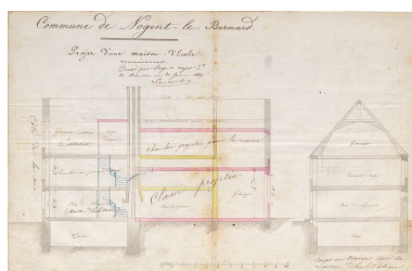
Projet d'appropriation d'une maison en mairie-école : coupes, 1849 Phot. Yves Guillotin, Autr. Laurent IVR52_20107202055NUCAB
