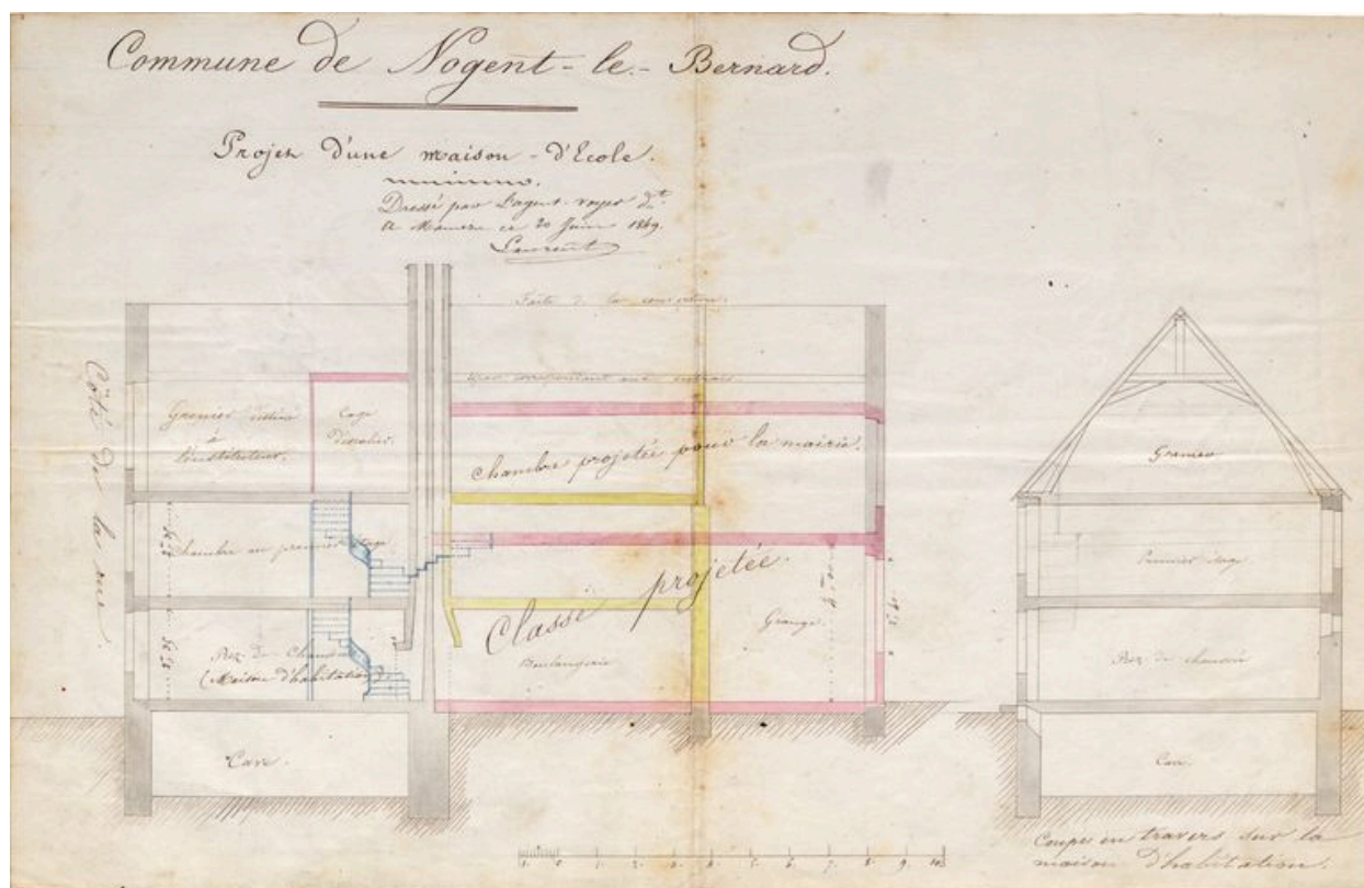
Projet d'appropriation d'une maison en mairie-école : coupes, 1849
