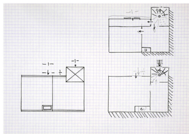
Plans schématiques (toitures, RdC, 1er étage), établis lors du pré- inventaire de 1979 (nord à droite). Croquis, feutre sur papier 21x297 cm. Autr. Dominique Eraud, Phot. Bruno Rousseau IVR52_20104902178NUCA
