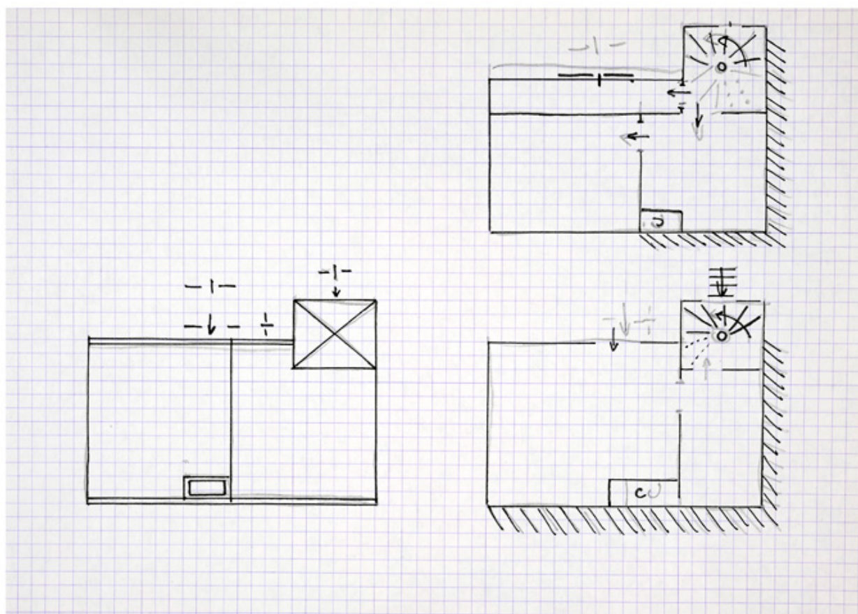
Plans schématiques (toitures, RdC, 1er étage), établis lors du pré-inventaire de 1979 (nord à droite). Croquis, feutre sur papier 21x297 cm.
