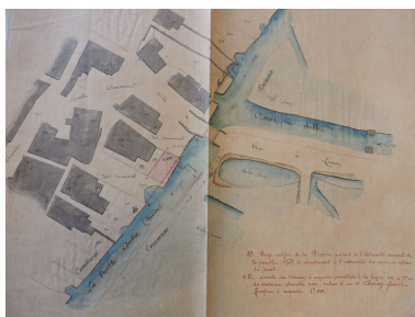
Plan d'agrandissement du port de la Grande Bernegoue, par l'ingénieur Espitallier, 26 mai 1868. Phot. Yannis (reproduction) Suire IVR52_20218501496NUCA
