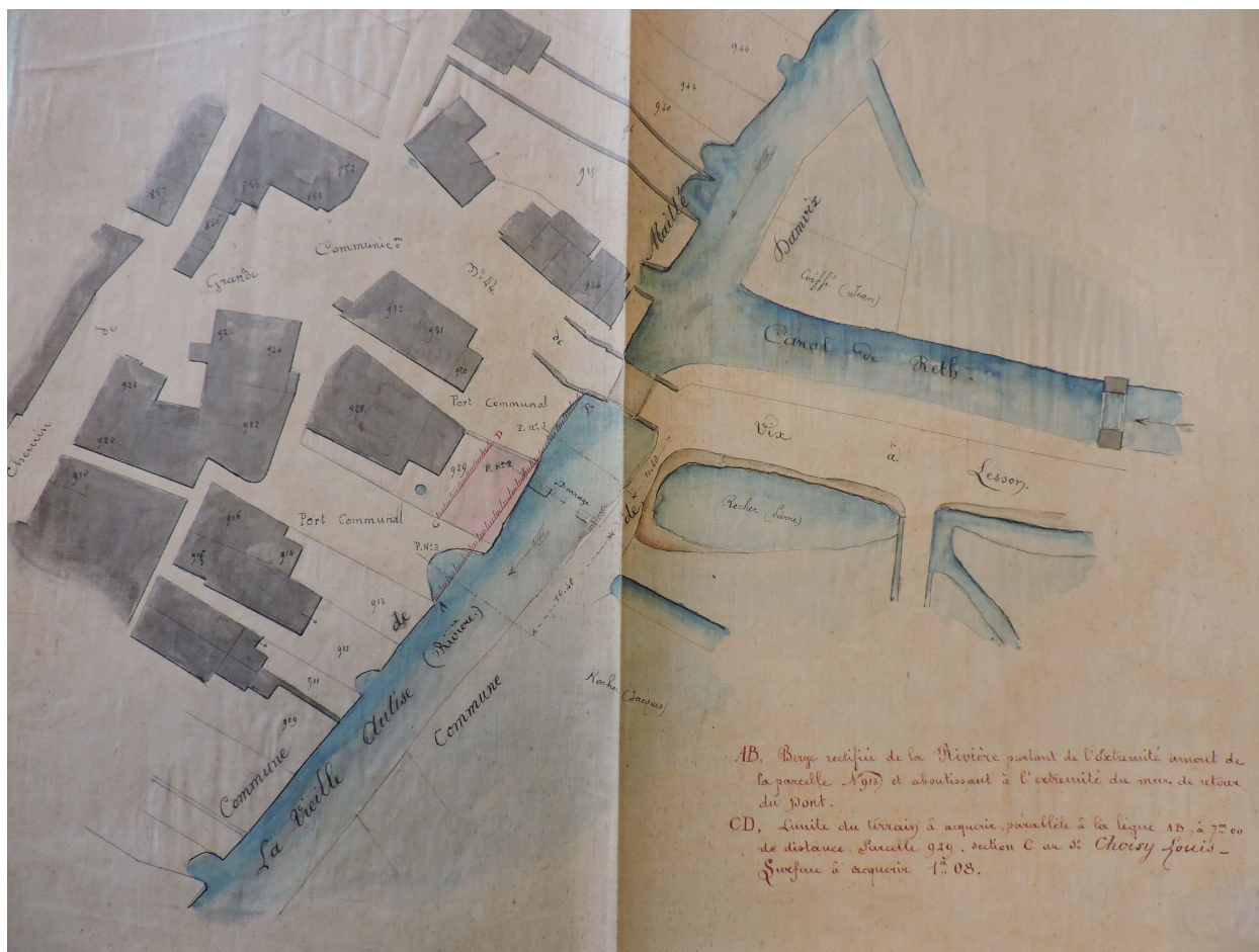
Plan d'agrandissement du port de la Grande Bernegoue, par l'ingénieur Espitallier, 26 mai 1868.
