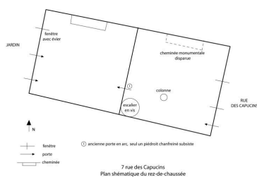
Plan schématique du rez-de-chaussée. Dess. Frédéric Dufrêche IVR52_20074403086NUCA
