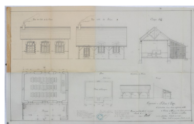
Construction d'une classe mixte, de water-closets et de préaux pour l'école primaire ; plans, élévations et coupes de la classe et du préau. Autr. Léopold Ridet, Phot. François Lasa IVR52_20035302875NUCA
