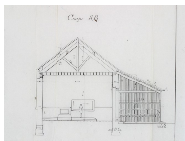
Construction d'une classe mixte, de water-closets et de préaux pour l'école primaire ; plans, élévations et coupes
