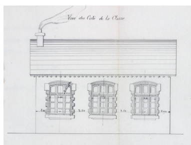
Construction d'une classe mixte, de water-closets et de préaux pour l'école primaire ; plans, élévations
