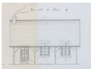
Construction d'une classe mixte, de water-closets et de préaux pour l'école primaire ; plans,
