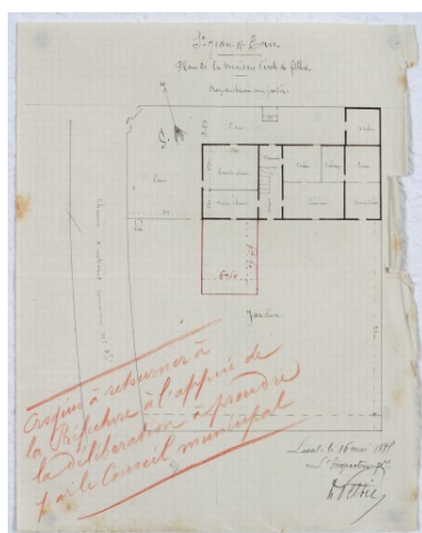
Plan de l'école et de son extension projetée (non réalisée) en 1885. Le document est signé par l'inspecteur primaire. Phot. François Lasa IVR52_20035302881NUCA
