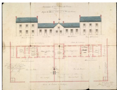
Projet de 1879, plan et élévation. Repro. Morgane Acou-Le Noan IVR52_20205300440NUCA
