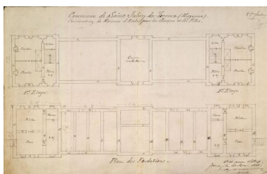
Projet de 1881, plan. Repro. Morgane Acou-Le Noan IVR52_20205300446NUCA
