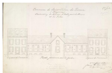
Projet de 1881, élévation. Repro. Morgane Acou-Le Noan IVR52_20205300447NUCA
