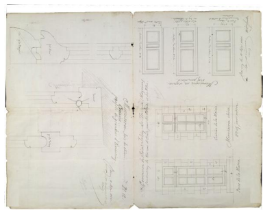
Projet de 1881, menuiseries. Repro. Morgane Acou-Le Noan IVR52_20205300452NUCA
