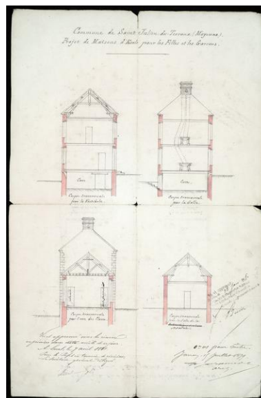
Projet de 1879, coupe. Repro. Morgane Acou-Le Noan IVR52_20205300442NUCA
