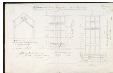
Projet de 1881, menuiseries des portes. Repro. Morgane Acou-Le Noan IVR52_20205300450NUCA
