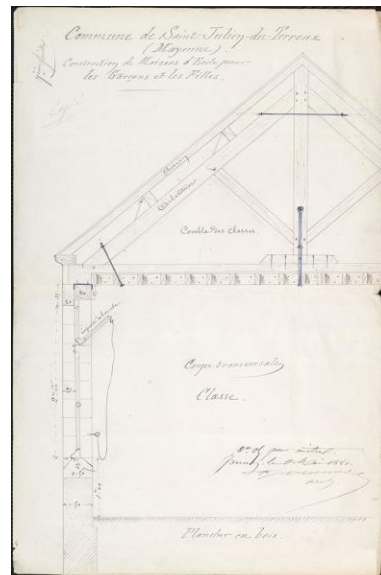
Projet de 1881, coupe de la charpente. Repro. Morgane Acou-Le Noan IVR52_20205300449NUCA
