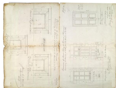
Projet de 1881, menuiseries. Repro. Morgane Acou-Le Noan IVR52_20205300451NUCA
