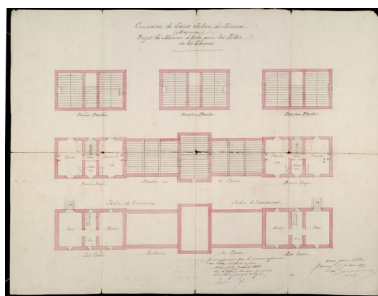
Projet de 1879, plan par niveau. Repro. Morgane Acou-Le Noan IVR52_20205300441NUCA
