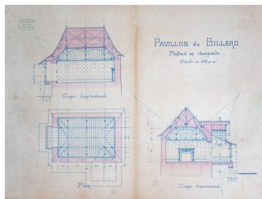
Les plans de la salle de billard par Louis Legrand, 1892. Autr. Louis Legrand, Phot. Pierre-Bernard Fourny IVR52_20235301381NUCA
