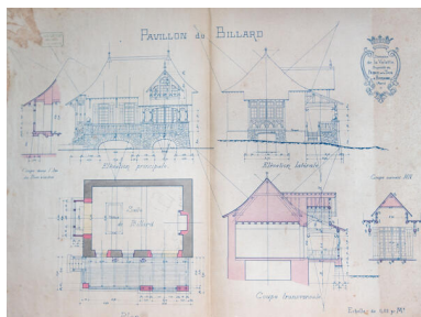
Les plans de la salle de billard par Louis Legrand, 1892. Autr. Louis Legrand, Phot. Pierre-Bernard Fourny IVR52_20235301374NUCA
