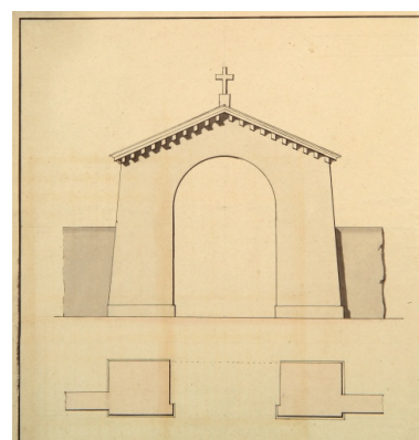
Projet de portail (détail) de l'entrepreneur Louis Michée. Autr. Louis Michée, Phot. Denis (reproduction) Pillet IVR52_20074400342NUCA
