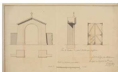
Projet de portail de l'entrepreneur Louis Michée. Autr. Louis Michée, Phot. Denis (reproduction) Pillet IVR52_20074400341NUCA
