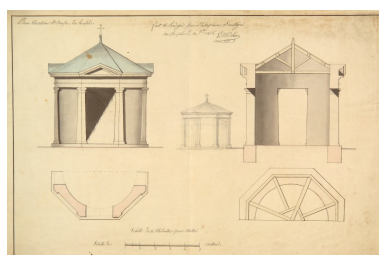
Projet de temple de l'entrepreneur Louis Michée. Autr. Louis Michée, Phot. Denis (reproduction) Pillet IVR52_20074400344NUCA
