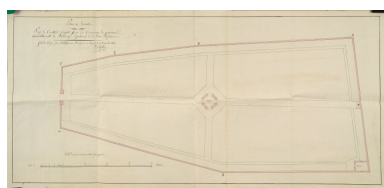
Avant projet de l'entrepreneur Louis Michée. Autr. Louis Michée, Phot. Denis (reproduction) Pillet IVR52_20074400340NUCA
