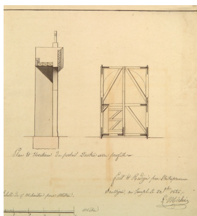
Projet de portail (détail) de l'entrepreneur Louis Michée. Autr. Louis Michée, Phot. Denis (reproduction) Pillet IVR52_20074400343NUCA
