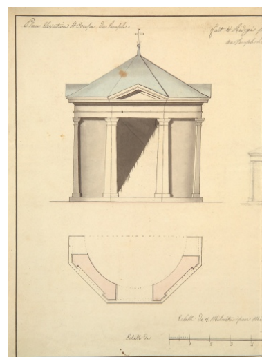
Projet de temple (détail) de l'entrepreneur Louis Michée. Autr. Louis Michée, Phot. Denis (reproduction) Pillet IVR52_20074400345NUCA
