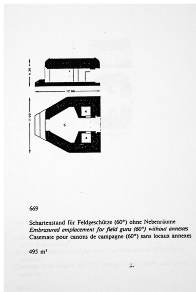
Plan d'une casemate de type H 669 pour canon de 105 mm. Phot. Denis (reproduction) Pillet IVR52_20074401174NUCA
